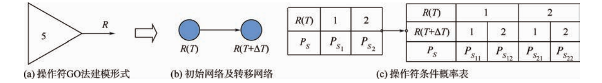
图 6 第 5 类操作符及对应动态贝叶斯网络
