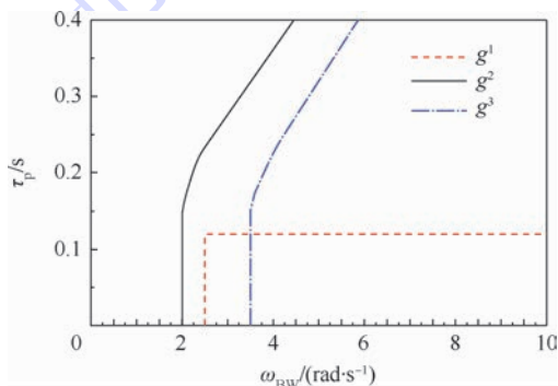
图 4 带宽一级飞行品质边界线
