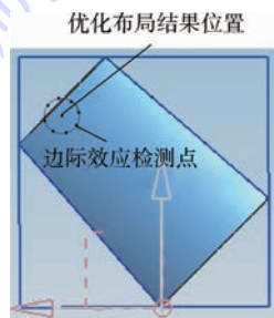
图 13 边界效应约束方法示意图
