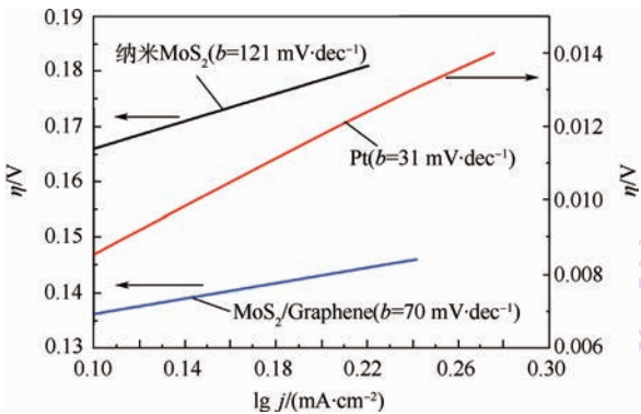
图 7 纳米 MoS 2 、MoS 2 /Graphene 以及 Pt 催化剂的塔菲尔曲线 Fig. 7 Tafel plots for nano MoS 2 , MoS 2 /Graphene and Pt catalysts
