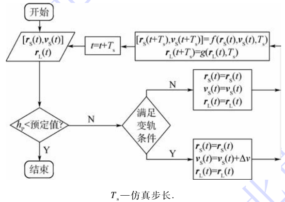
图 6 连续脉冲变轨仿真计算流程图
