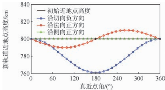
图 4 3 个速度分量变化的影响程度对比
