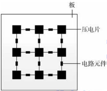
图1 压电网络板 Fig.1 Piezo electro mechanical-plate
