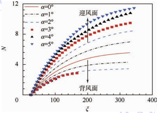
图 10 eN 方法的 N 值曲线
