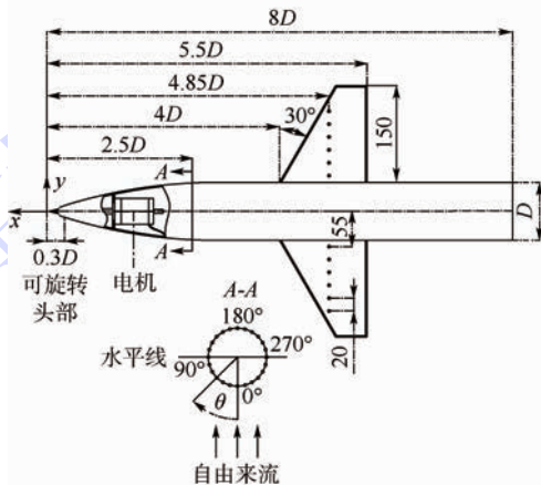
(b) 实验模型尺寸图 (尺寸单位: mm)
