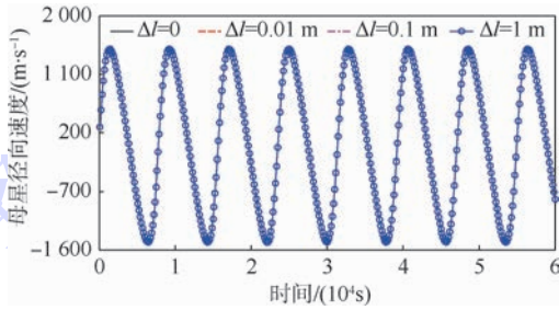
图 7 CCPTS 质心径向速度随时间变化关系
