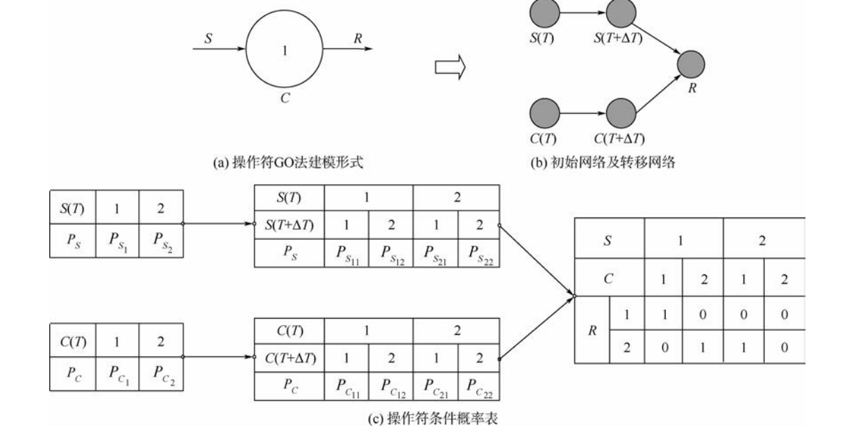
图 5 第 1 类操作符及对应动态贝叶斯网络
