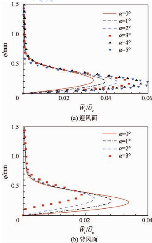
图 7 在 \xi=100 处横流速度剖面 Fig. 7 Profile of crossflow velocity at \xi=100
