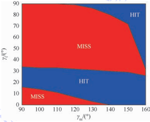
图8 FTGC 的拦截区域
