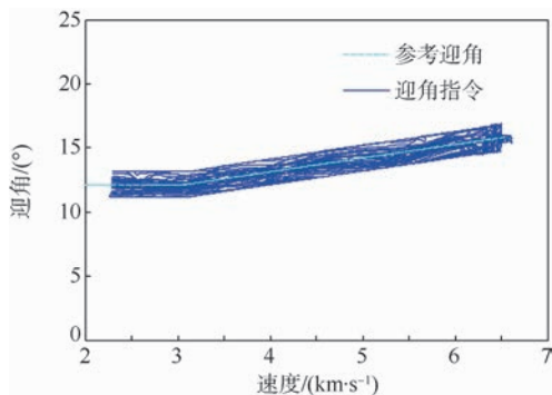
图 7 迎角控制历程
