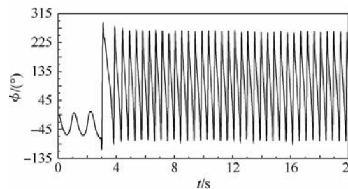
(c) 振荡发散时间历程( \alpha=45^\circ )
