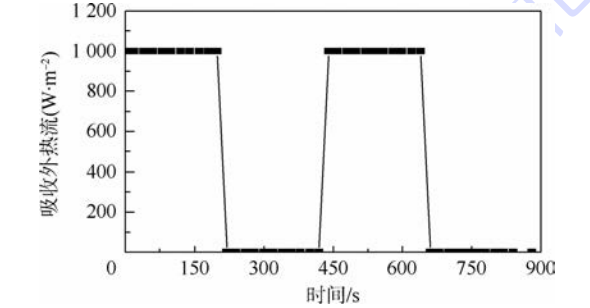
图 4 数值试验 2 的吸收外热流曲线 Fig. 4 Absorbed external heat flux curve of numerical experiment 2
