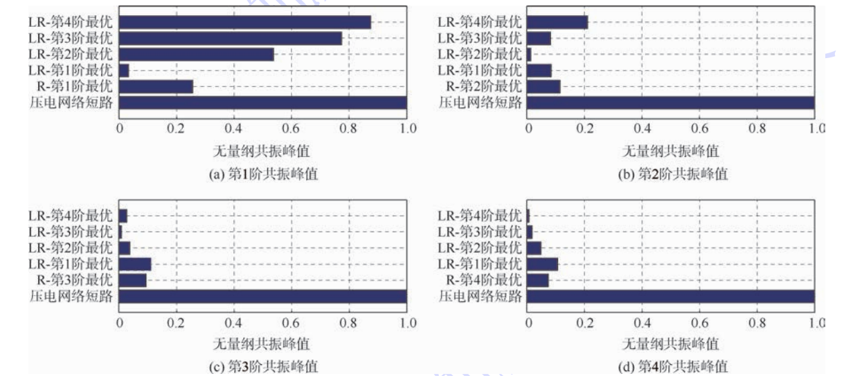
图 14 各类最优电学参数对共振峰值的影响的比较 Fig. 14 Comparison among influence of optimal circuit parameters on resonance peak value
