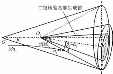
图 3 第 2 级压缩基准流场
