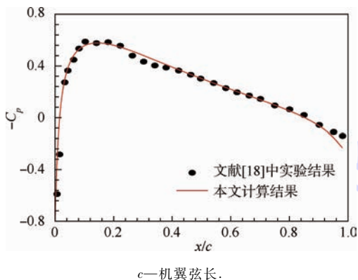
图 3 压力系数沿弦长方向分布
