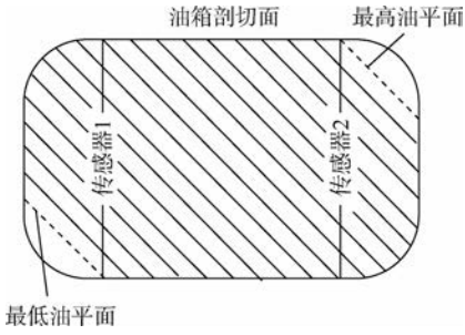
图 6 最大燃油可测区示意图
