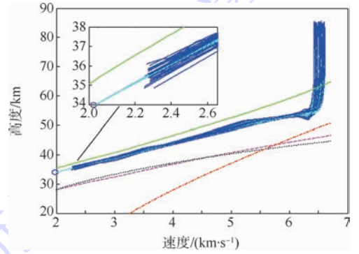
图 5 速度-高度剖面跟踪 Fig. 5 Trajectory tracking in velocity-altitude profile
