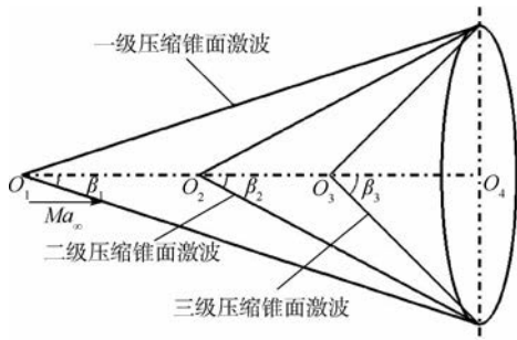
图 1 三级压缩锥形激波的设计预期流场
