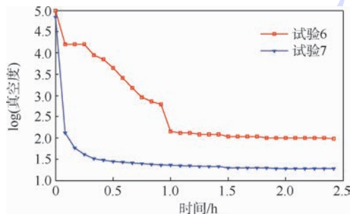
图11 密度对真空度的影响
