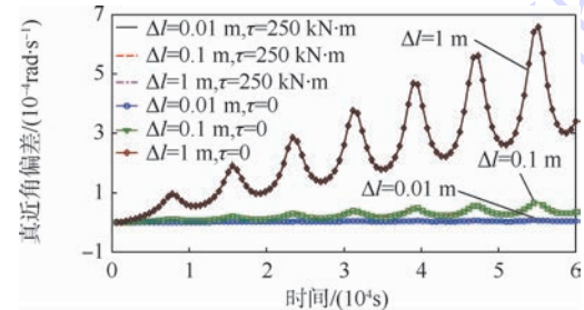
图 13 系绳长度偏差对真近角的影响 Fig. 13 Influence of tether length deviation on true anomaly angular
