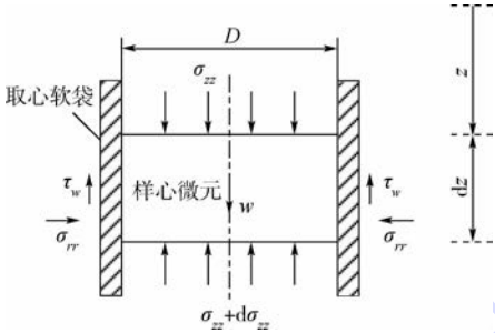
图 4 土体 I 微元 Fig.4 Element in Soil I
