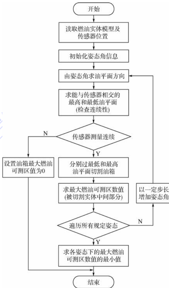
图 11 油箱最大燃油可测区数值计算流程图
