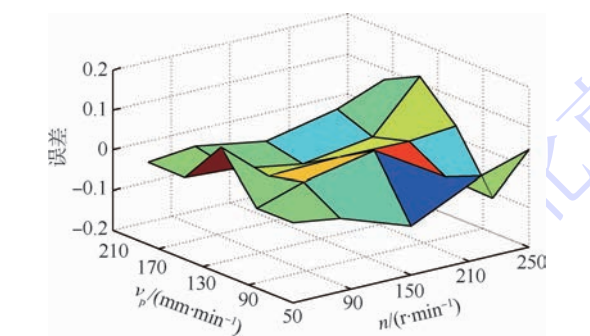
图 15 取心率计算误差 Fig. 15 Calculation error of coring rate
