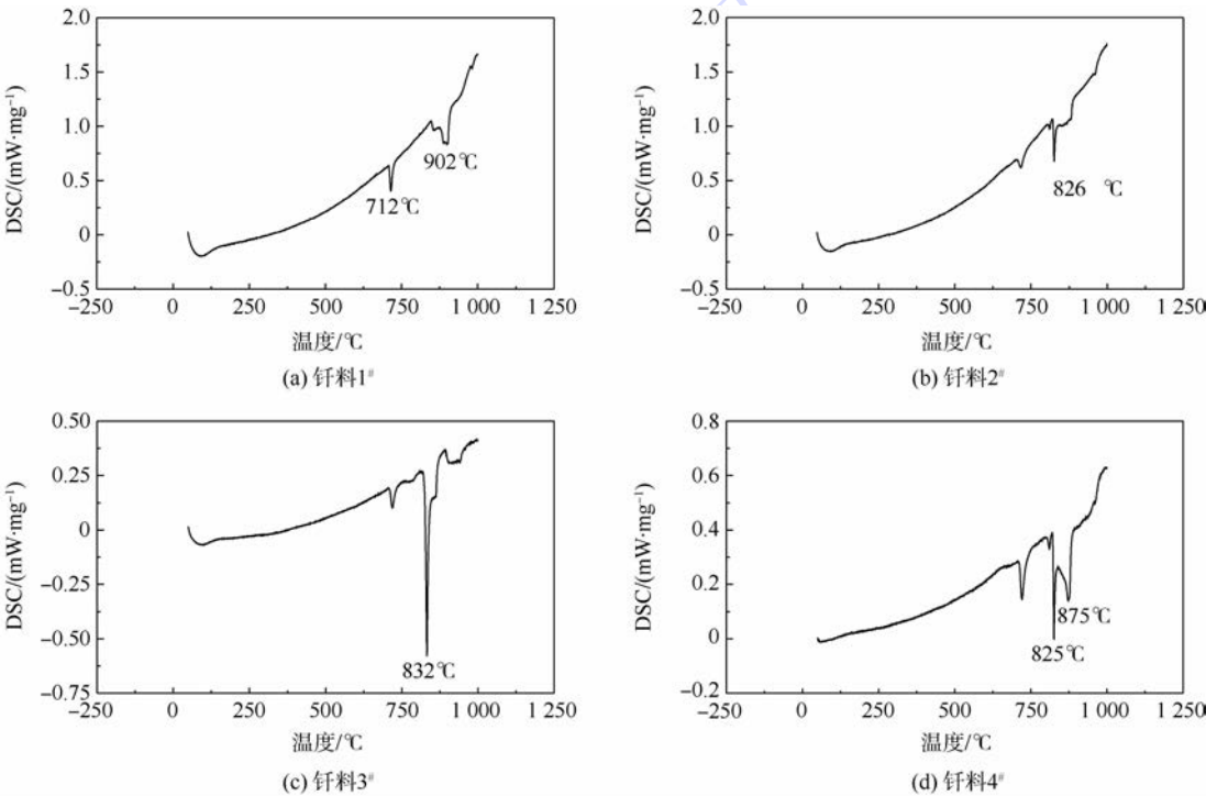
图 2 钎料的 DSC 曲线 Fig. 2 DSC curves of brazing filler metals
