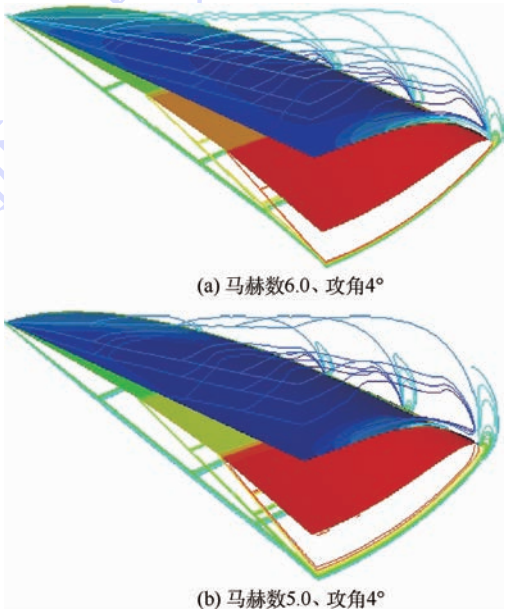
图 12 三级压缩锥导乘波体非设计状态等压线图
