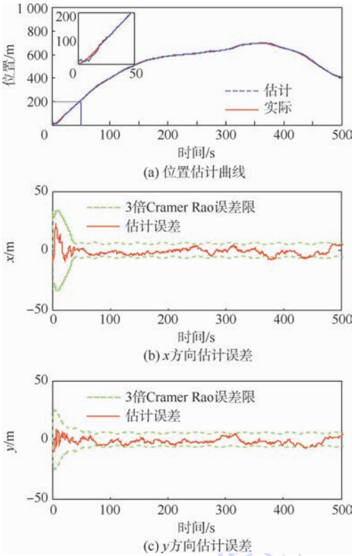
图5 运动目标位置估计
