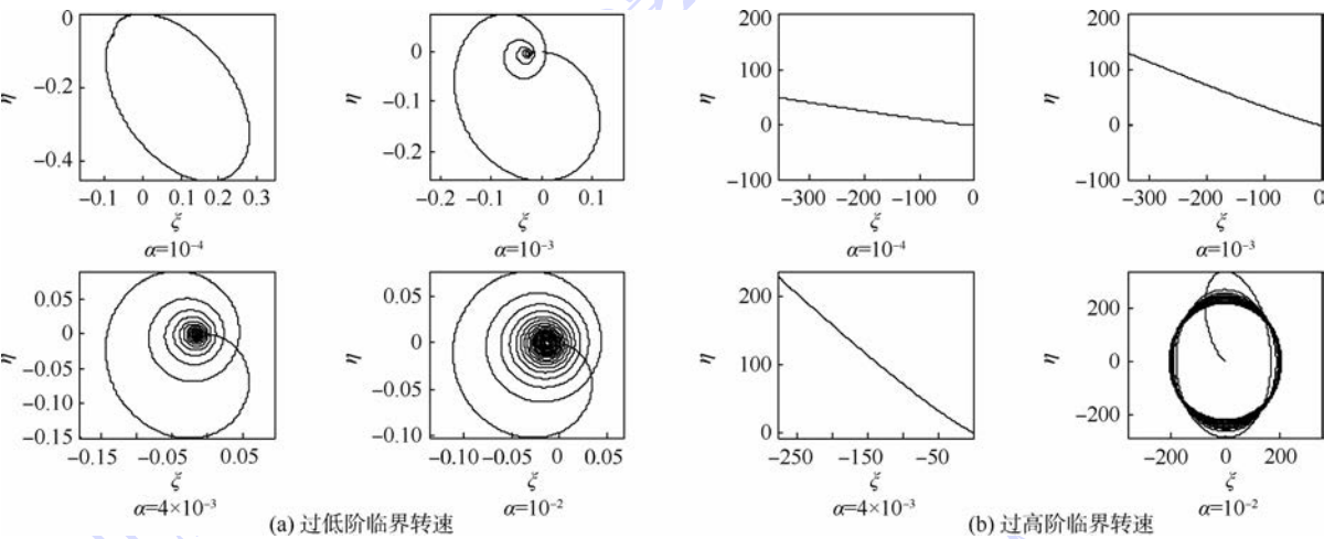
图 12 不对称厚盘转子过低阶及高阶临界转速盘偏角矢尖轨迹
