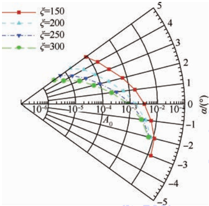
图 12 初始扰动幅值 A_0 随攻角的变化曲线
