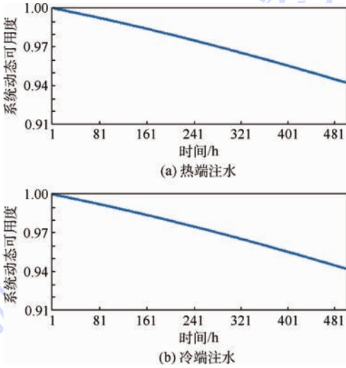
图 13 核电站高压注水系统动态可用度
