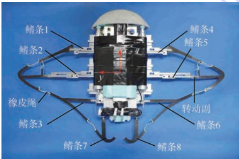
图 2 物理样机 Fig. 2 Physical prototype
