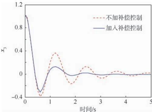
图 3 x_3 控制效果
