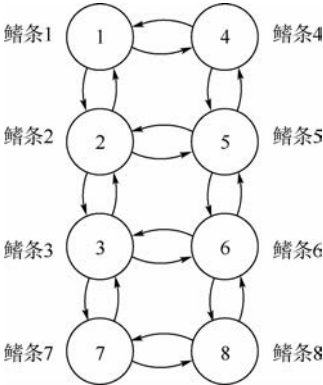
图 8 CPG 网络结构示意图 Fig. 8 CPG network structure schematic
