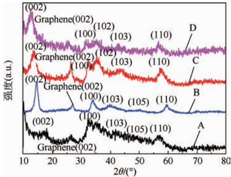
A, B, C, D—水热合成过程中 \text{Na}_2\text{MoO}_4 \cdot 2\text{H}_2\text{O} 的浓度为 1 mmol, \text{NH}_2\text{CSNH}_2 的浓度分别为 5、6、7 和 8 mmol 时所制备得到的 \text{MoS}_2/\text{Graphene} .
