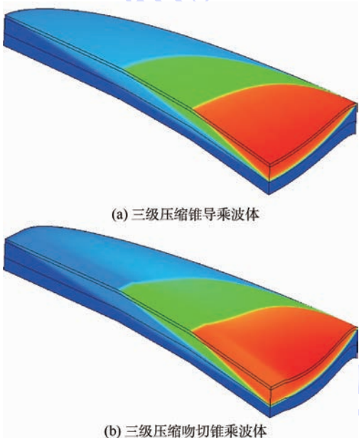
图 9 三级压缩乘波体激波结构图 Fig. 9 Shockwave structural diagram of TSC waverider
