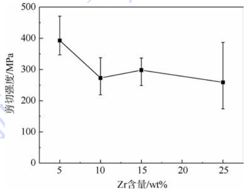
图 6 钎焊接头的剪切强度 Fig. 6 Shear strength of brazed joints
