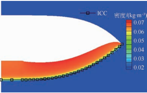
图 10 三级压缩吻切锥乘波体底部截面密度云图 Fig. 10 Density contours of TSC osculating cone waverider's bottom section
