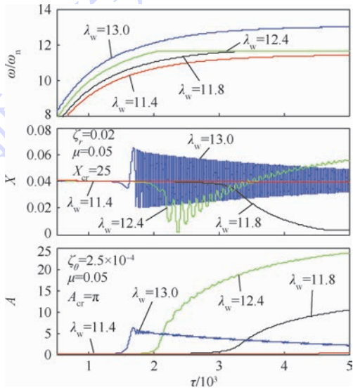
图 22 对称厚盘转子定功率过高阶临界转速时随时间变化的瞬态振动曲线
