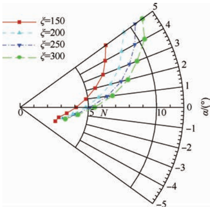
图 11 N 值随攻角的变化曲线
