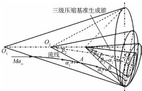
图 4 第 3 级压缩基准流场
