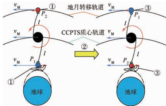
图 2 CCPTS 进行载荷转移过程示意图
