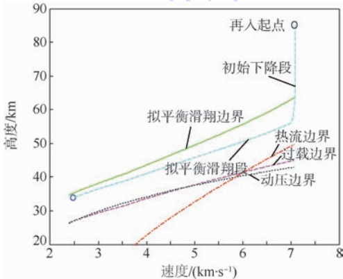
图 1 再入轨迹的构成 Fig. 1 Composition of entry trajectory
