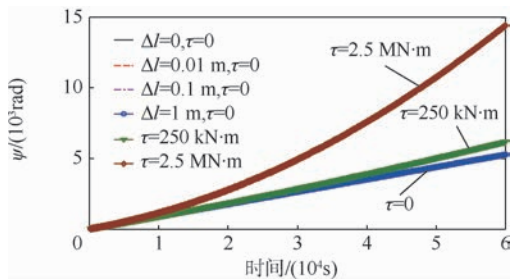
图 9 系绳与重力方向夹角随时间变化关系
