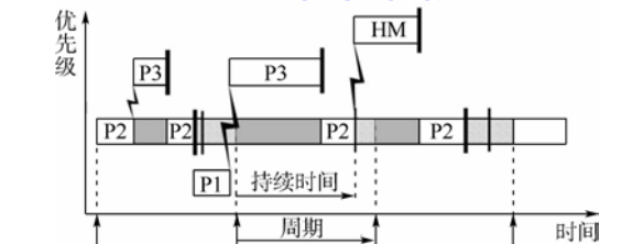
图 9 进程调度 Fig.9 Process schedule
