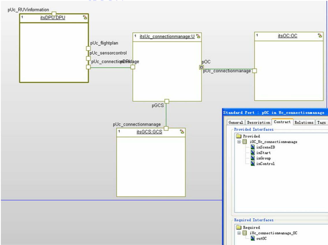
图 4 内部块图
