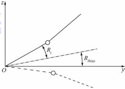
图 7 鳍条摆动中心线定义 Fig. 7 Definition of fin oscillating center line
