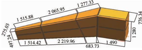
图 4 燃油实体模型外形尺寸(单位:mm)
