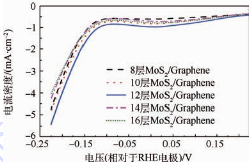
(b) 旋涂不同层数的 \text{MoS}_2/\text{Graphene} 催化剂的电催化活性的比较
