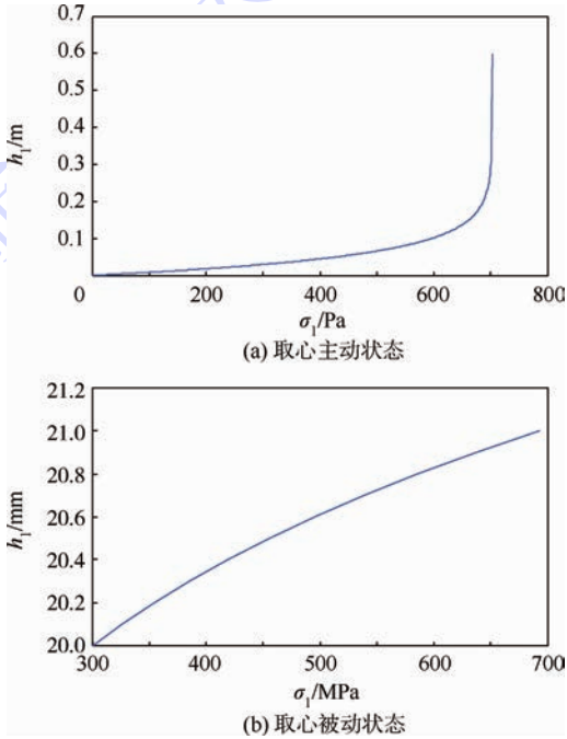
图 6 土体 I 主被动状态下的底面应力 Fig.6 Bottom stress of soil I in active and passive states
