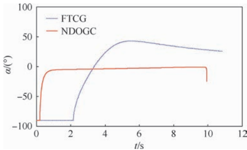
图3 导弹和非机动目标的攻角变化
