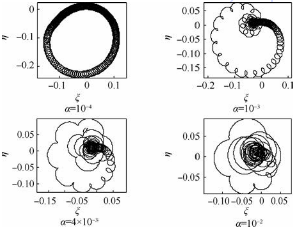
图 9 计重力过低阶临界转速时盘偏角矢尖在旋转坐标中的轨迹
