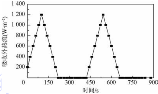
图 1 数值试验 1 的吸收外热流曲线
