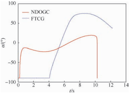
图5 导弹和机动目标的攻角变化
