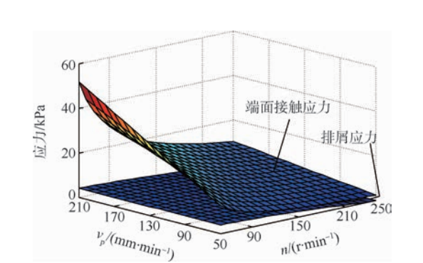
图 17 外伸管钻头取心应力组成 Fig. 17 Coring stress composition of extended tube drill bit
