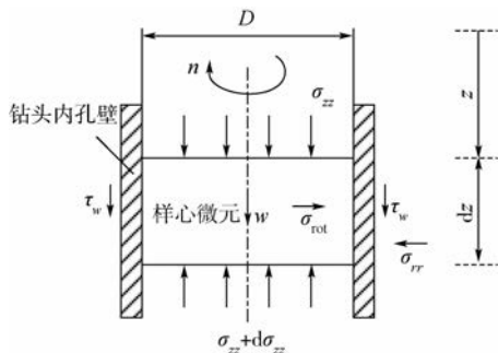
图 7 土体 II 微元
