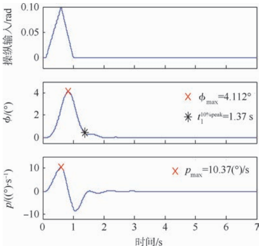
图 12 滚转通道尖峰输入响应
