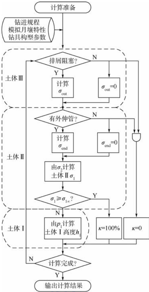
图 10 取心模型的计算流程
