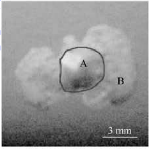
(d) 钎料4 # (25wt% Zr)
