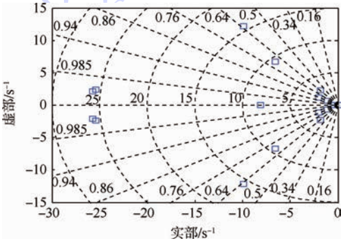
图 6 闭环系统特征值 Fig. 6 Eigenvalues of closed-loop system
