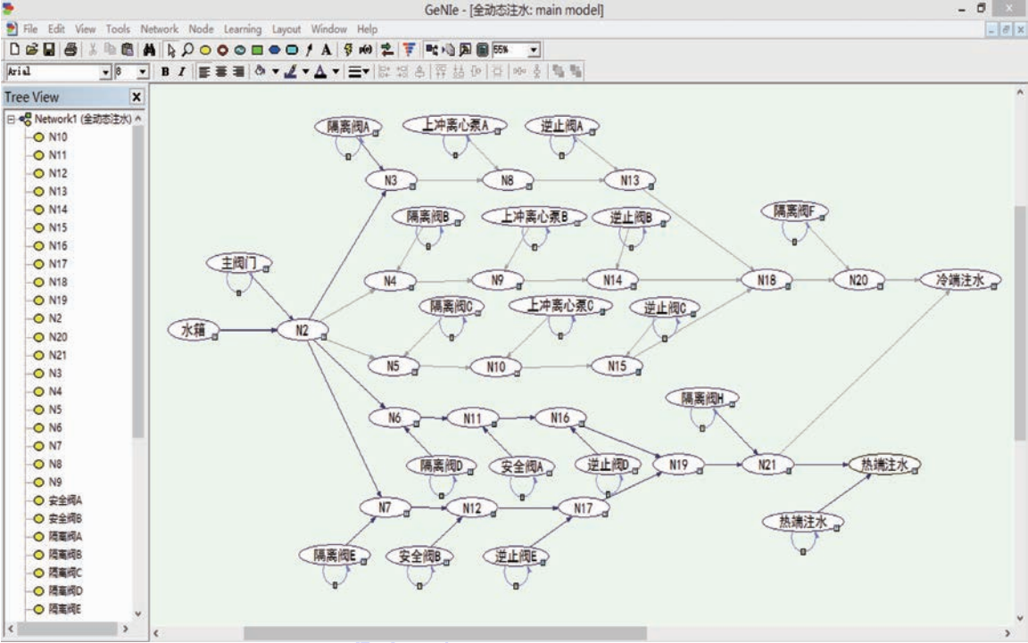
图 12 核电站高压注水系统动态贝叶斯网络转移图
