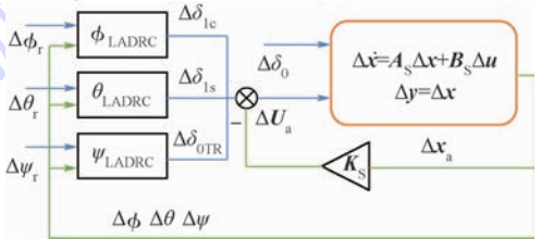
图 3 带反馈内回路的态度控制器
