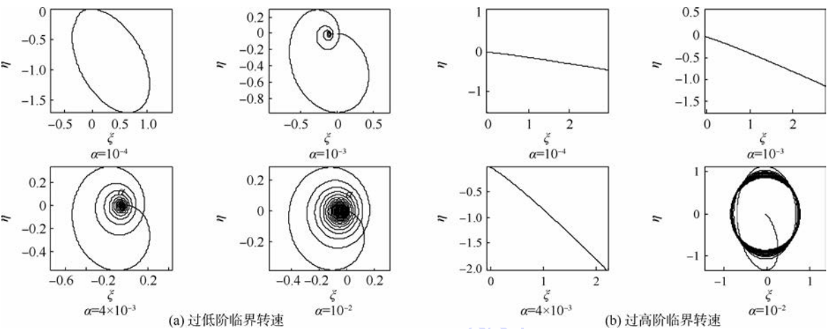
图 11 不对称厚盘转子过低阶及高阶临界转速形心轨迹
