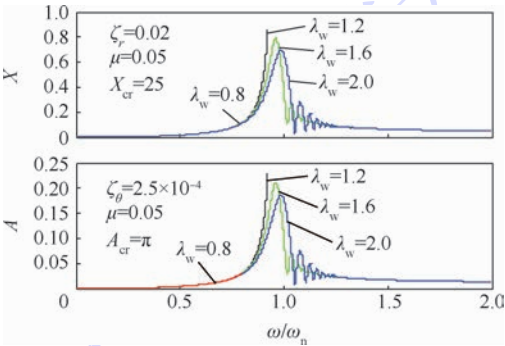
图 14 低阶临界转速附近工作的对称厚盘转子随转速的瞬态振动曲线
