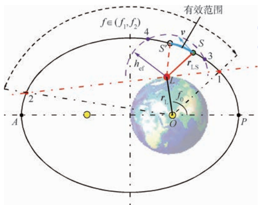
图 5 确定变轨区域示意图
