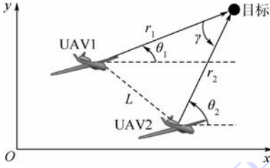
图 1 角度测量下的协同目标观测
