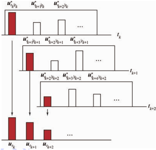
图 2 滚动时域控制原理图 Fig. 2 RHC schematic
