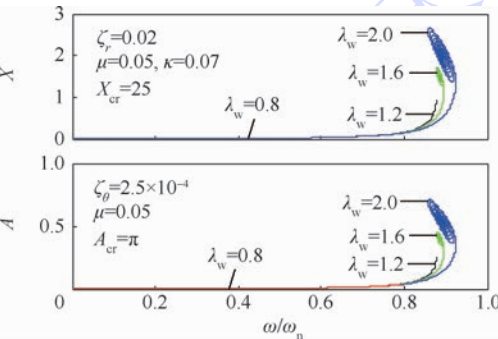
图 20 低阶临界转速附近工作的非对称 ( \kappa=0.07 ) 厚盘转子随时间的瞬态振动曲线
