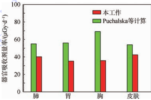
图 10 计算的航天员受银河宇宙线照射的器官吸收剂量率与 PHITS 计算结果比较
