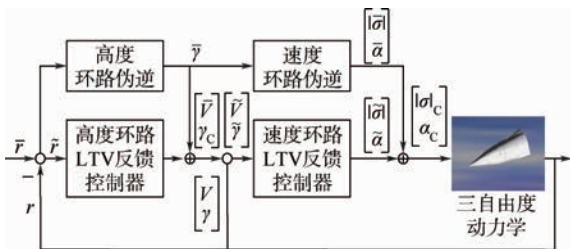
图 3 制导回路 TLC 结构图 Fig. 3 Configuration of TLC in guidance loop
