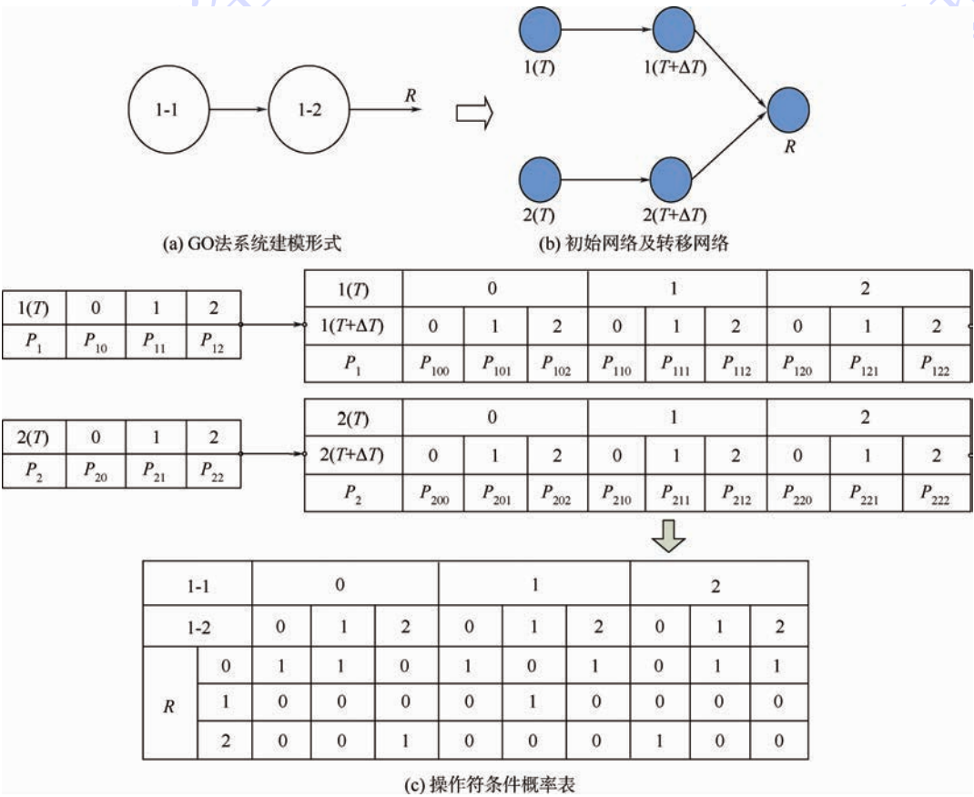
图 8 操作符之间的停工相关
