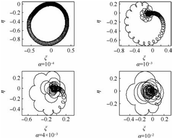
图 8 计重力过低阶临界转速的厚盘转子形心在旋转坐标中的轨迹
