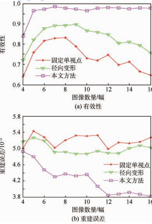
图 6 不同方法在不同输入图像数量条件下的性能比较 Fig. 6 Performance comparison among different methods with varying number of input images
