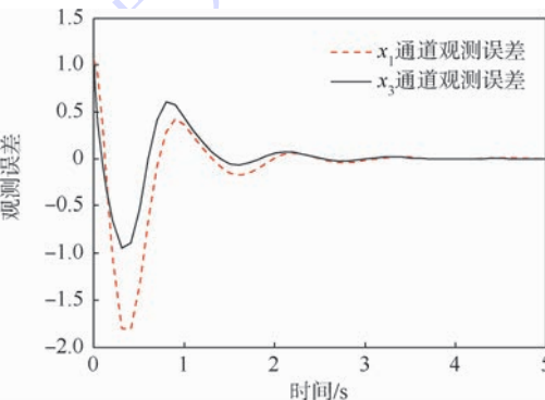
图 4 模糊神经网络观测误差
