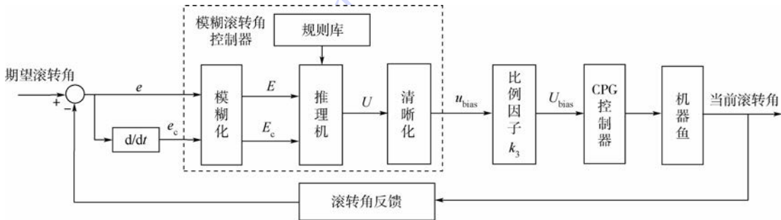
图 9 基于 CPG 的模糊控制器结构
