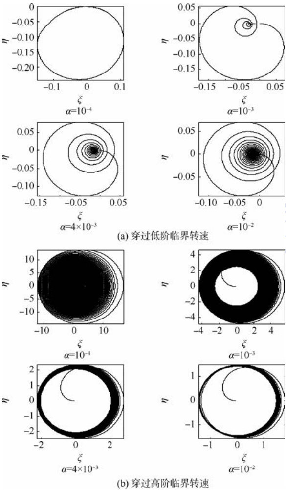
图 6 穿过低阶及高阶临界转速时盘偏角矢尖在旋转坐标系中的轨迹( \mu=0.05 )
