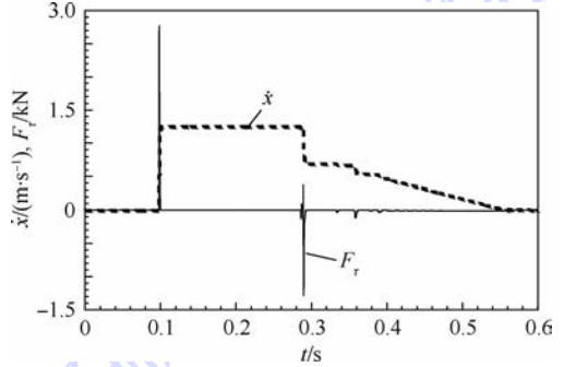
图 6 \dot{x} 和 F_{\tau} 的时间历程图
