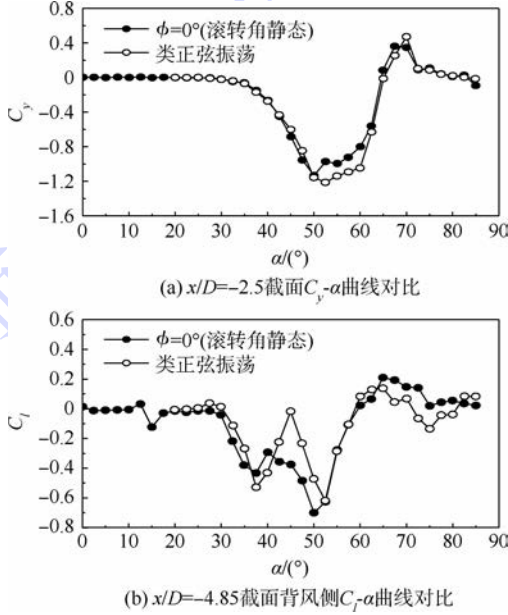
图 9 攻角拉起类正弦振荡与单独攻角拉起(ϕ=0°)两种情形下 C y -α 及 C l -α 曲线对比(ω=40(°)/s)
