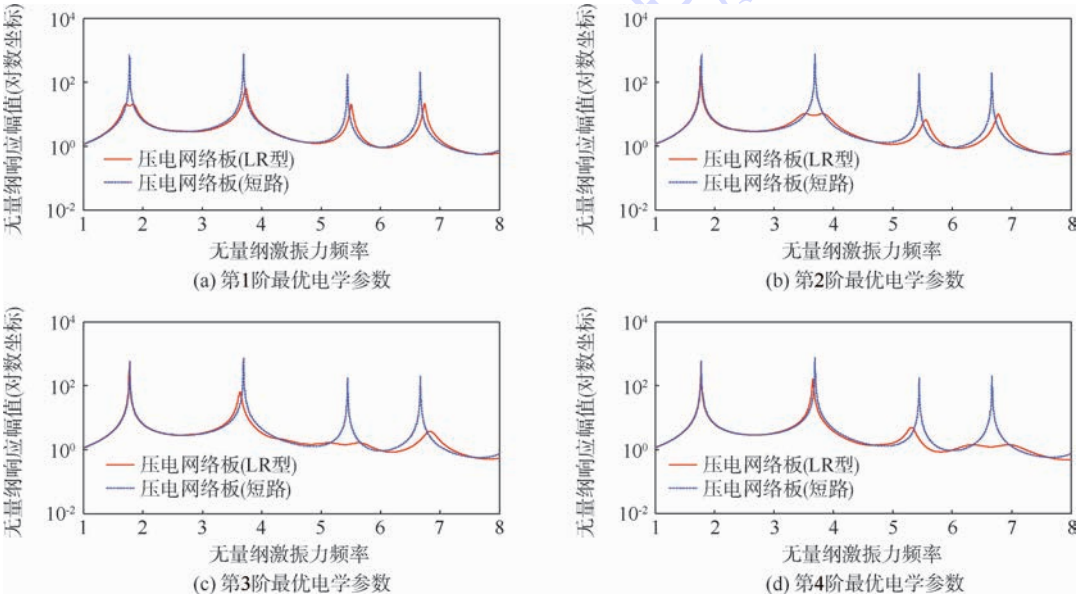
图 12 LR-PEM 振动控制效果
