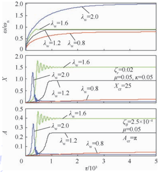
图 16 低阶临界转速附近工作的非对称 ( \kappa=0.05 ) 厚盘转子随时间的瞬态振动曲线
