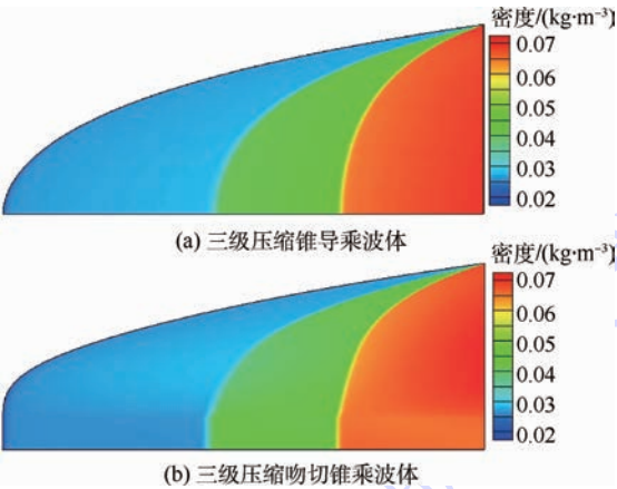
图 8 三级压缩乘波体下表面密度云图 Fig. 8 Density contours of TSC waverider's lower surface
