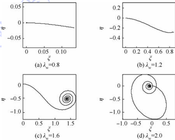
图 18 非对称 ( \kappa=0.05 ) 厚盘转子在低阶临界转速附近振动的形心轨迹
