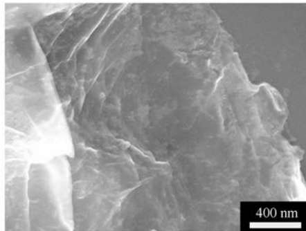
(b) GO的SEM照片
