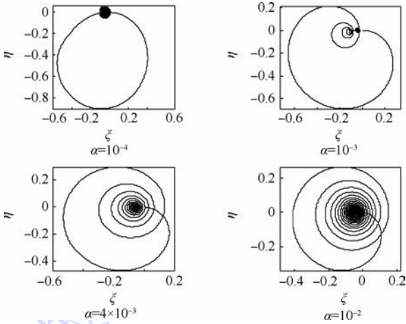
图 4 整个加速过程形心在旋转坐标系中的轨迹( \mu = 0.05 )
