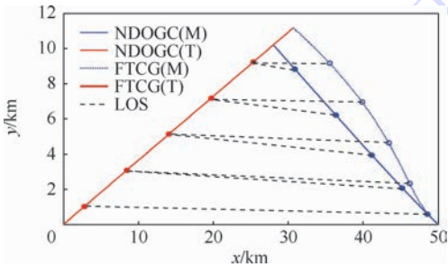
图2 导弹和非机动目标相对运动轨迹
