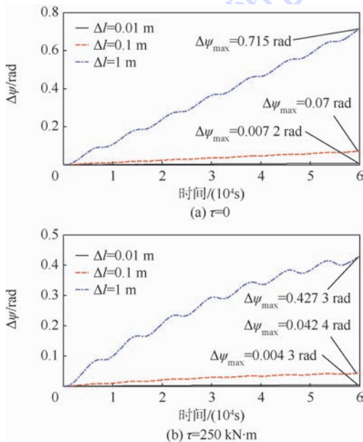
图 10 系绳长度偏差对系绳与重力方向之间夹角的影响
