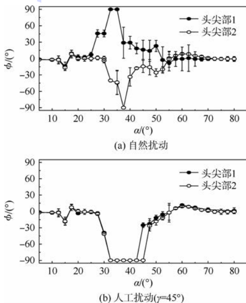
图 2 外形相同的两个头尖部下,摇摆运动平衡位置及均方差随攻角的变化规律( \omega = 0(^\circ)/s )
