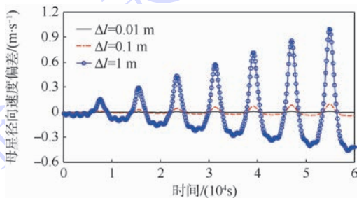
图 8 系绳长度偏差对 CCPTS 质心径向速度的影响
