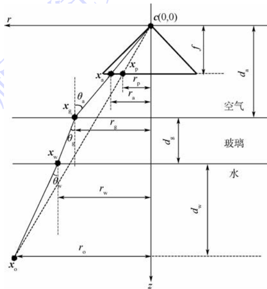
图 2 水下相机成像过程二维示意图
