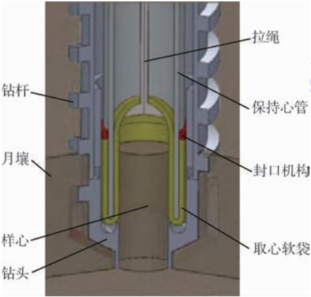
图 1 软袋钻取采样机构组成
