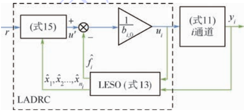
图 2 LADRC 控制器框图
