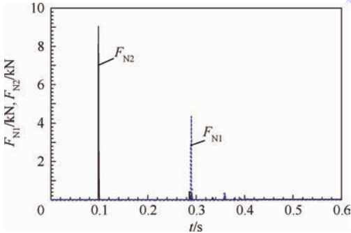
图 3 F_{N1} 和 F_{N2} 的时间历程图
