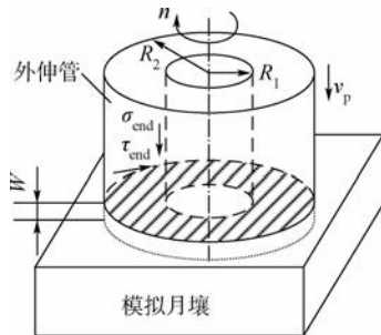
图 8 圆管端面与土体面接触
