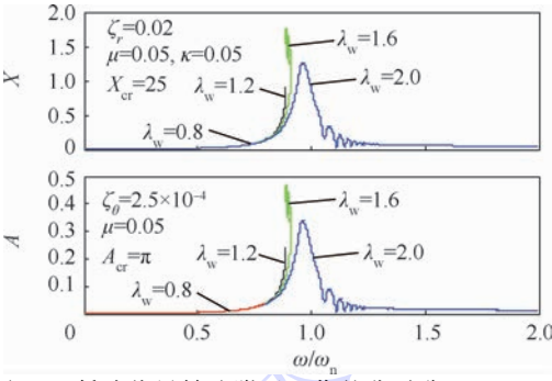
图 17 低阶临界转速附近工作的非对称 ( \kappa=0.05 ) 厚盘转子随转速的瞬态振动曲线
