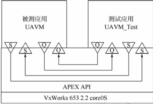
图 10 应用测试框图
