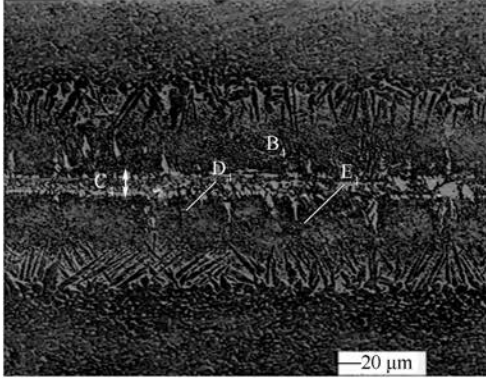
(d) 25wt% Zr
