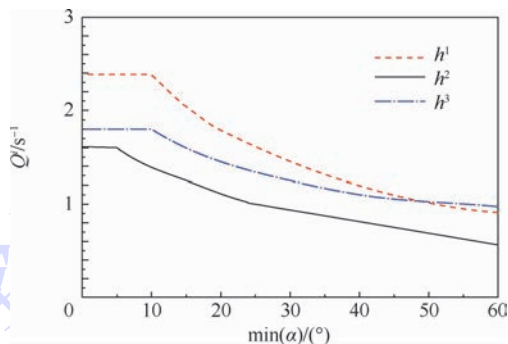
图 5 快捷性一级飞行品质边界线
