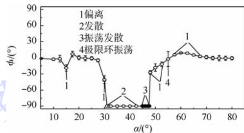
(a) 摇摆运动随攻角变化规律
