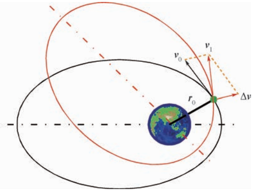
图 2 脉冲变轨示意图
