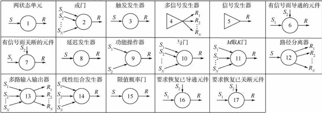
图 1 GO 法操作符类型 Fig. 1 Type of GO methodology operators
