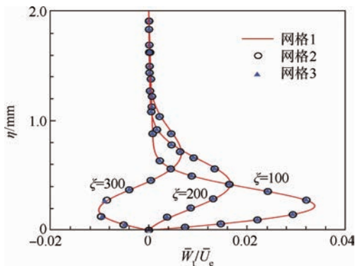
图 4 横流速度剖面
