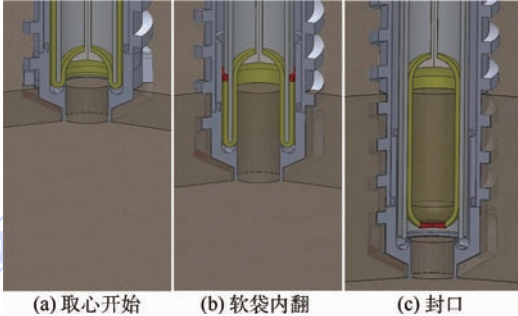
图 2 软袋取心工作过程
