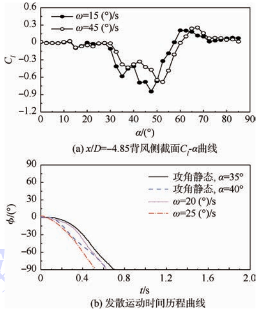
图 8 拉起速度对机翼背风侧截面滚转力矩系数和摇摆时间历程曲线的影响
