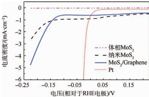
(a) 不同电催化剂(体相 \text{MoS}_2 、纳米 \text{MoS}_2 、 \text{MoS}_2/\text{Graphene} 以及 Pt)的电催化制氢性能的比较
