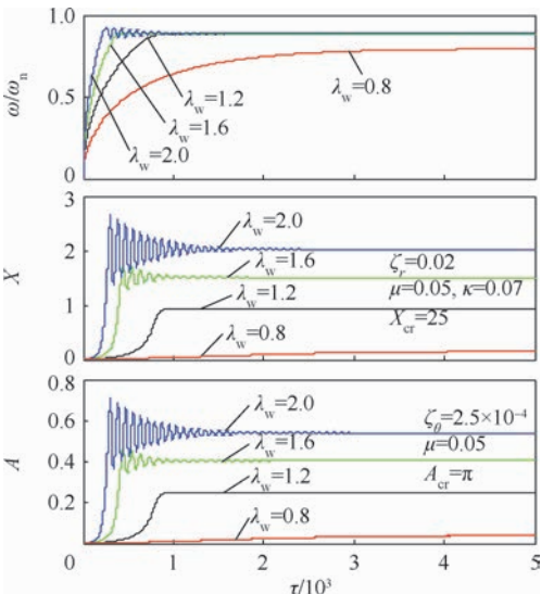
图 19 低阶临界转速附近工作的非对称 ( \kappa=0.07 ) 厚盘转子随时间的瞬态振动曲线
