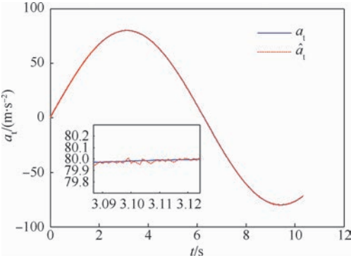
图6 目标加速度的估计
