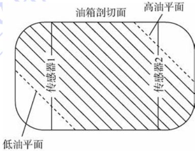
图 5 燃油可测区示意图
