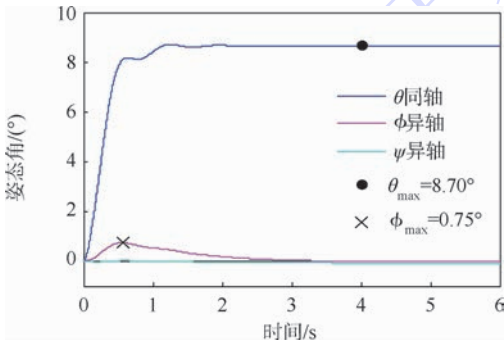
图 11 俯仰通道阶跃输入下的耦合
