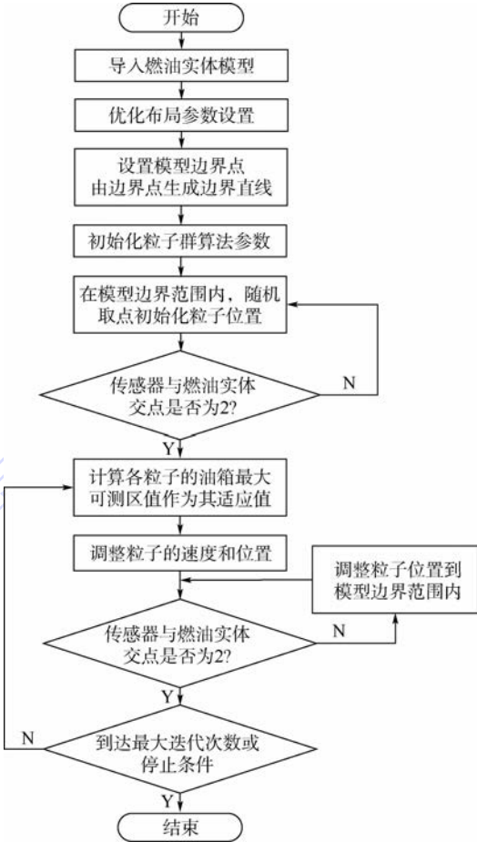
图 15 传感器优化布局的流程
