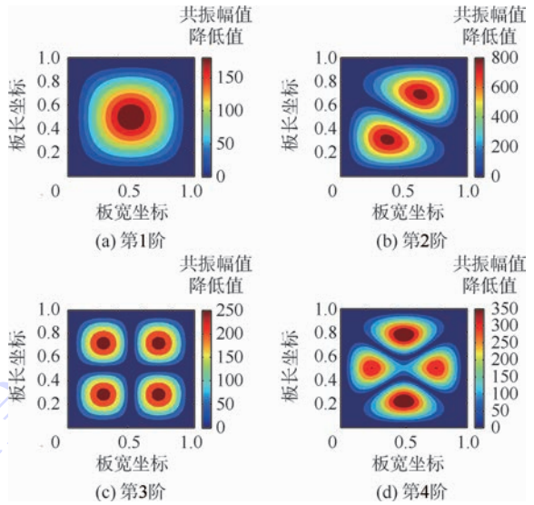
图 13 LR-PEM 振动抑制效果云图 Fig. 13 Contour of vibration suppression effect (LR-PEM)
