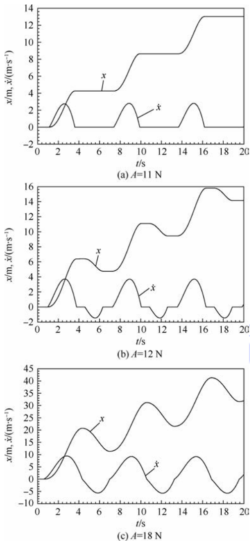
图 7 当 A = 11, 12, 18 N 时 x 和 \dot{x} 的时间历程图
