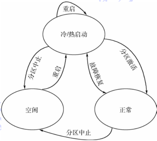
图 7 分区工作模式转换 Fig. 7 Partition working modes transform
