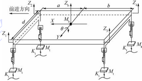
M_b —车身簧载质量; Z_b —车身质心位移; d —轴距; M_t —轮胎质量; K_t —轮胎刚度。
