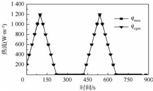
图 3 数值试验 1 的吸收外热流反演值与真实值比较
