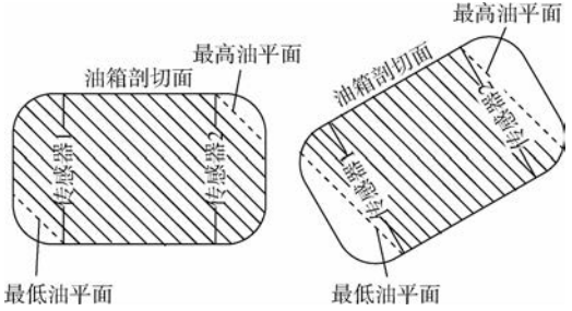
图 8 最大燃油可测区与飞行姿态的关系
