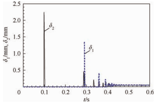
图 4 \delta_1 和 \delta_2 的时间历程图
