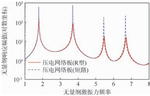
图 7 R-PEM 振动控制效果
