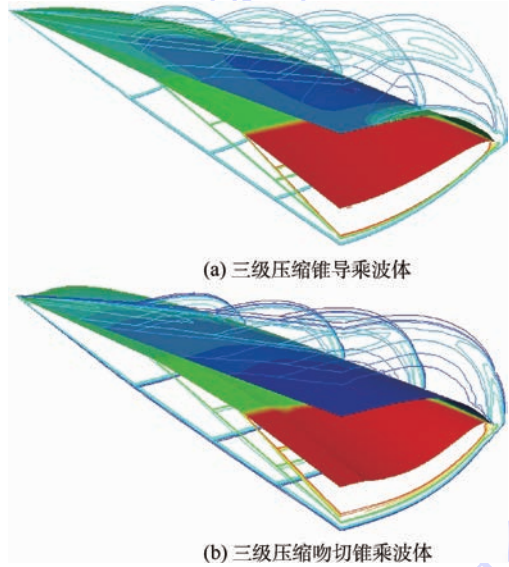
图 11 三级压缩乘波体等压线图
