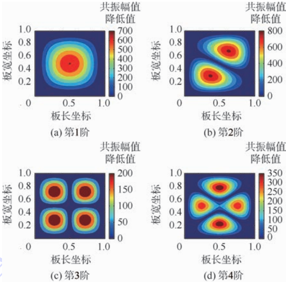
图 8 R-PEM 振动抑制效果云图
