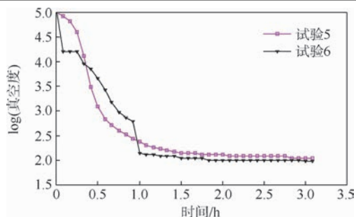
图9 样品量对真空度的影响
