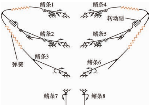
图 1 机构简图 Fig. 1 Mechanism schematic
