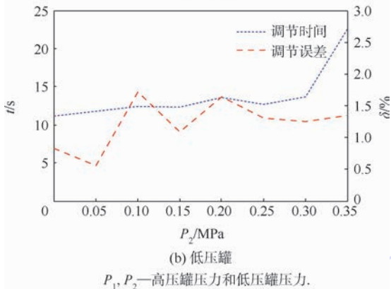
图 10 高压罐和低压罐不同初始气压对车身高度调节的影响
