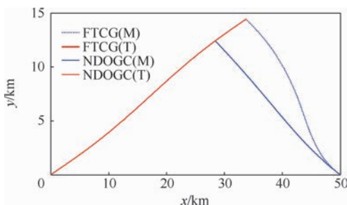
图4 导弹和机动目标相对运动轨迹
