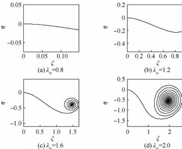
图 21 低阶临界转速附近工作的非对称 ( \kappa=0.07 ) 厚盘转子瞬态振动的形心轨迹
