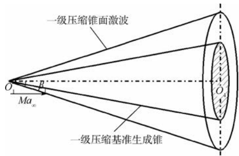
图 2 第 1 级压缩基准流场
