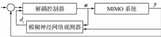
图 1 闭环系统结构 Fig. 1 Closed-loop system structure
