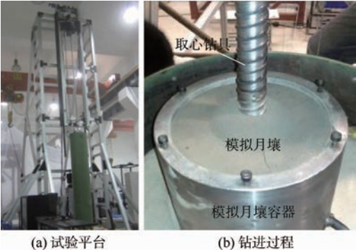
图 11 模拟月壤钻进取心试验及其平台
