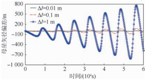
图 6 系绳长度偏差对 CCPTS 质心矢径的影响
