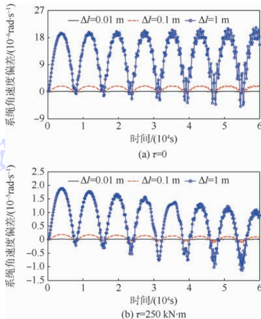
图 11 系绳长度偏差对系绳旋转角速度的影响
