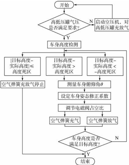
图 2 车身高度控制流程图
