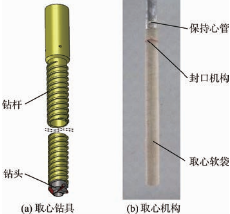
图 13 中空取心钻具
