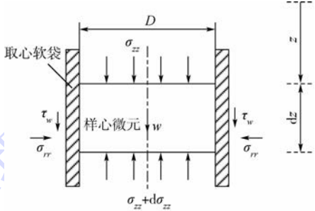
图 5 土体 I 微元向上运动 Fig.5 Upward movement of element in Soil I
