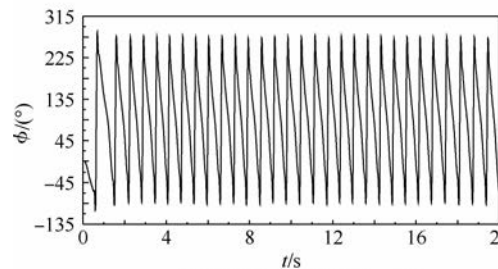
(b) 发散运动时间历程( \alpha=40^\circ )
