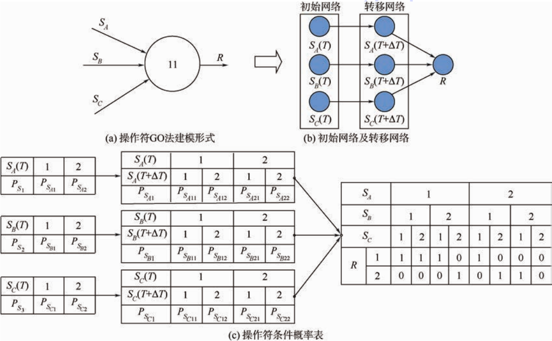
图 4 第 11 类操作符及对应动态贝叶斯网络
