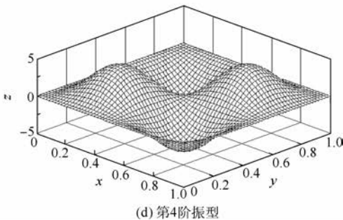
图5 四边固支板前4阶振型
