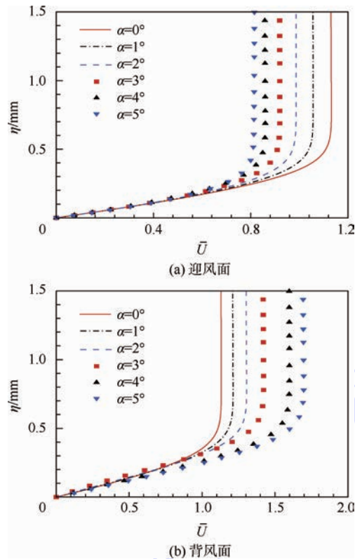
图 6 在 \xi=100 处的流向速度 \bar{U} 剖面 Fig. 6 Profile of flow velocity \bar{U} at \xi=100
