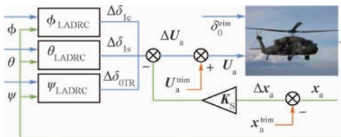
图 15 非线性动力学的姿态控制器
