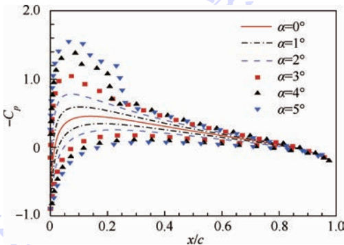
图 5 不同攻角下的压力系数
