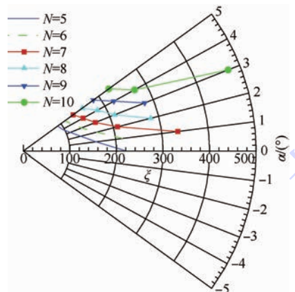
图 13 转捩位置 \xi 随攻角的变化曲线
