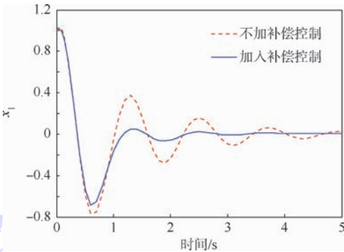
图 2 x_1 控制效果
