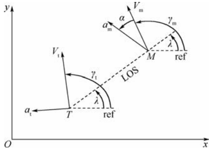
图 1 弹目拦截几何
