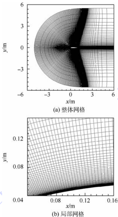
图 2 计算网格示意图
