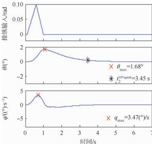
图 13 俯仰通道尖峰输入响应
