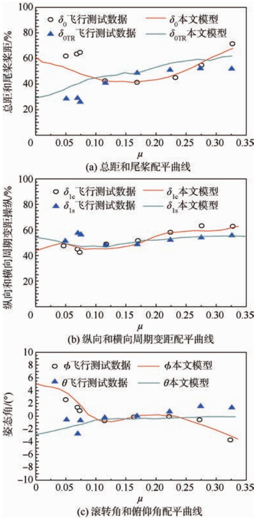
图 1 配平结果曲线 Fig. 1 Curves of trim results
