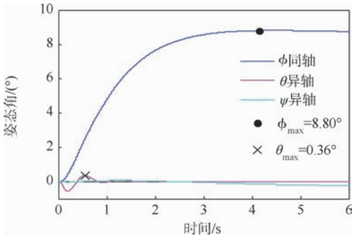
图 10 滚转通道阶跃输入下的耦合
