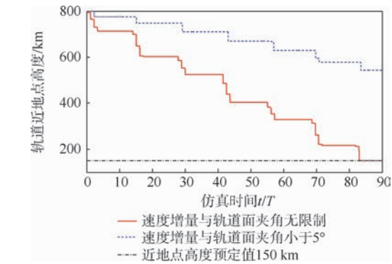
图 7 轨道近地点高度随时间变化曲线
