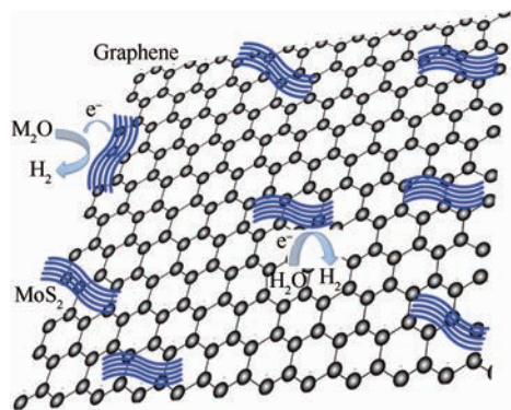
图 9 \text{MoS}_2/\text{Graphene} 复合催化剂里的电子转移机理图
