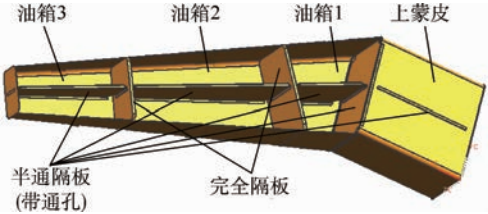
图 1 油箱物理模型示意图
