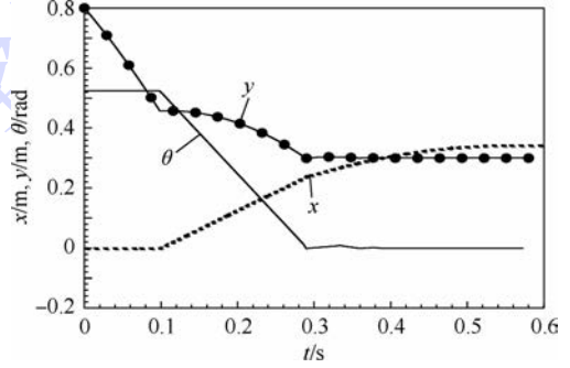
图 5 x 、 y 和 \theta 的时间历程图
