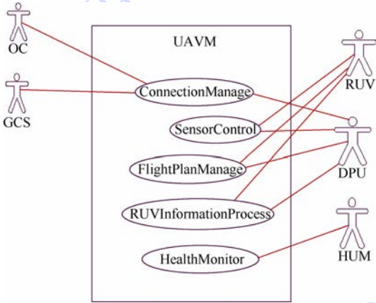
图 1 UAVM 系统用例图 Fig. 1 UAVM system use case diagram
