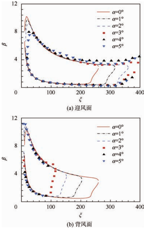
图 9 中性稳定曲线 ( \omega = 0 )
