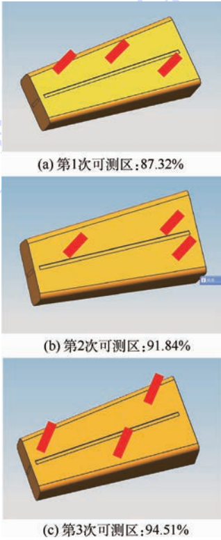
图 16 油箱 3 中布置 3 根传感器时的多次布局结果
