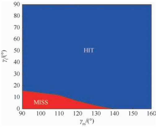
图9 NDOGC 的拦截区域
