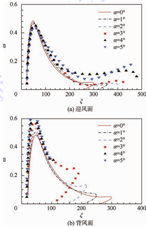
图 8 中性稳定曲线( \beta=3 ) Fig. 8 Neutral stability curves ( \beta=3 )
