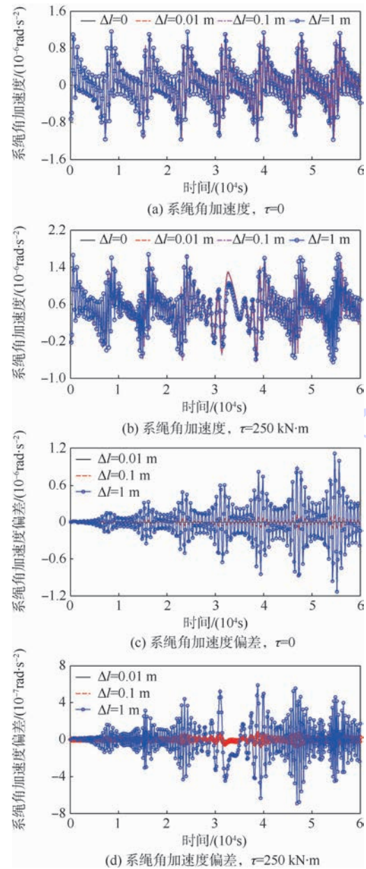
图 12 系绳长度偏差对系绳角加速度的影响 Fig. 12 Influence of tether length deviation on angular acceleration of tether
