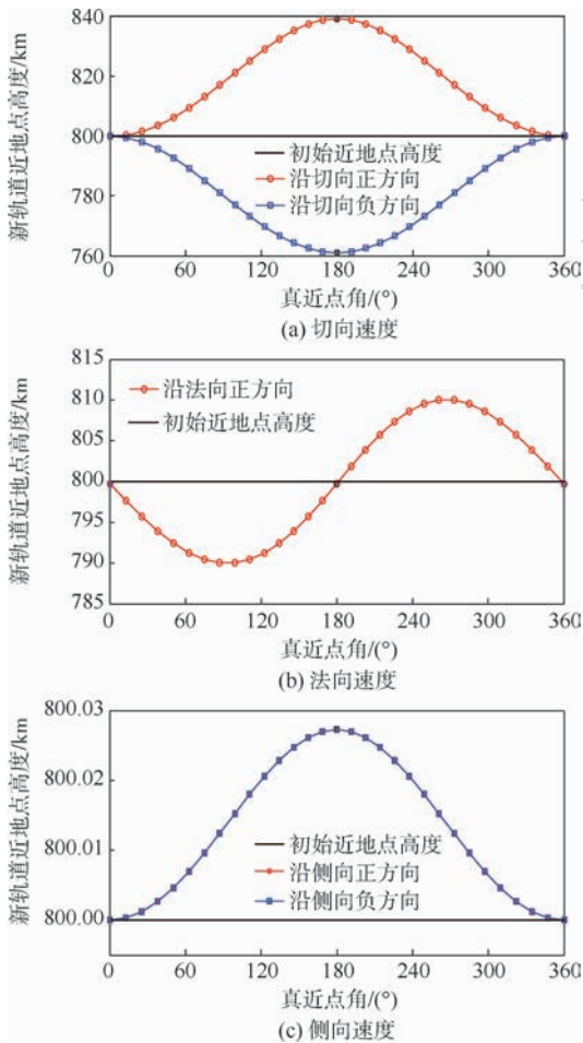
图 3 改变不同速度分量的降轨效果图
