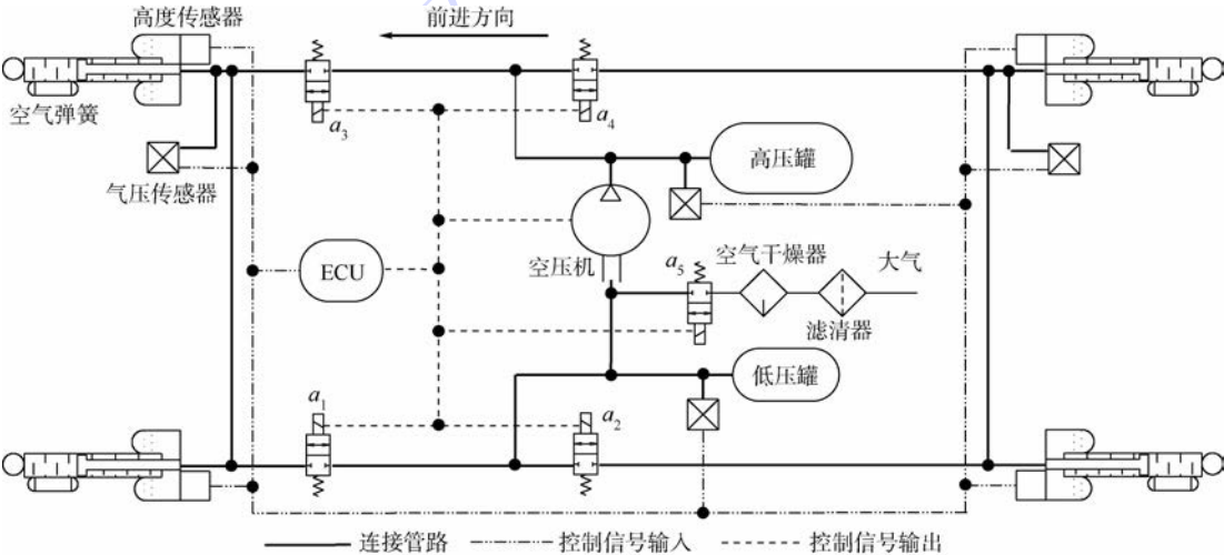
图 1 气路闭环横向互联空气悬架系统工作原理简图
