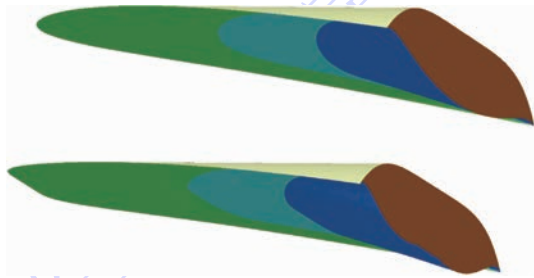
图 6 三级压缩锥导乘波体和吻切锥乘波体
