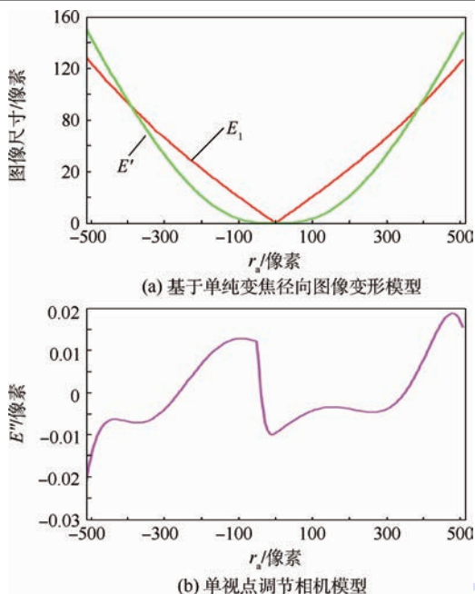
图3 不同相机模型的折射变形补偿能力
