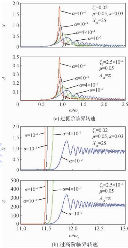
图 10 不对称厚盘转子过低阶及高阶临界转速的瞬态振动曲线
