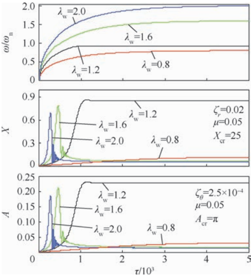
图 13 低阶临界转速附近工作的对称厚盘转子随时间的瞬态振动曲线
