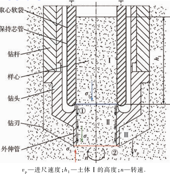
图 3 软袋取心准静态分析
