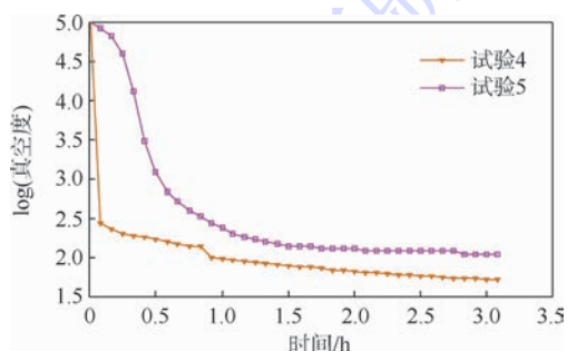
图10 含水量对真空度的影响
