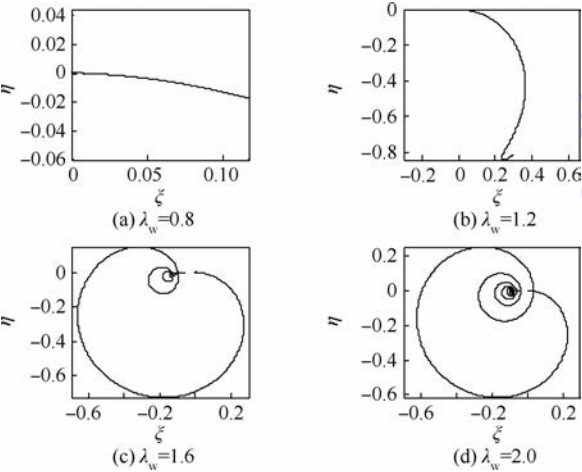
图 15 低阶临界转速附近工作的对称厚盘转子形心轨迹
