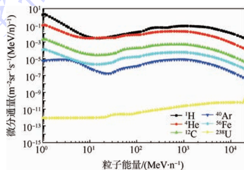
图4 国际空间站轨道银河宇宙线粒子 ( ^1\text{H} 、 ^4\text{He} 、 ^{12}\text{C} 、 ^{40}\text{Ar} 、 ^{56}\text{Fe} 和 ^{238}\text{U} ) 的能谱 Fig.4 Energy spectra of GCR particles ( ^1\text{H} 、 ^4\text{He} 、 ^{12}\text{C} 、 ^{40}\text{Ar} 、 ^{56}\text{Fe} 和 ^{238}\text{U} ) in ISS orbit
