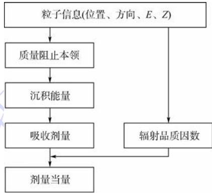
图 1 航天员器官剂量计算流程
