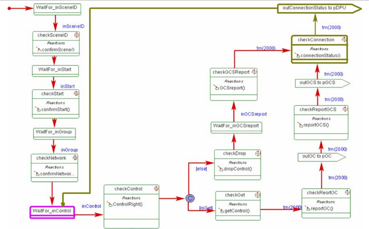
图 5 系统状态图
