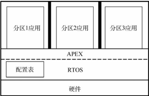
图 6 IMA 模块结构
