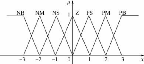
图 10 各语言变量的隶属度函数 Fig. 10 Membership function for each linguistic variable
