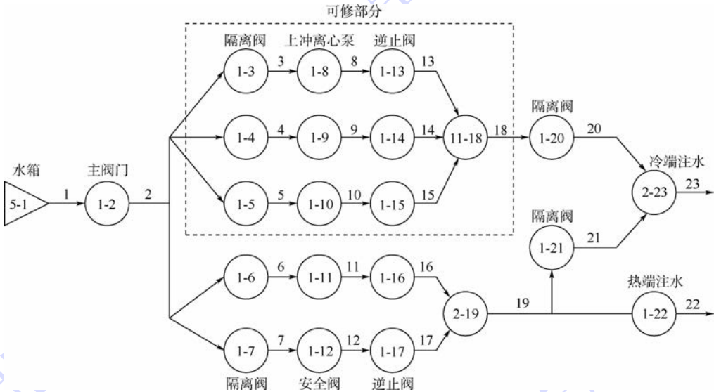
图 11 核电站高压注水系统 GO 图
