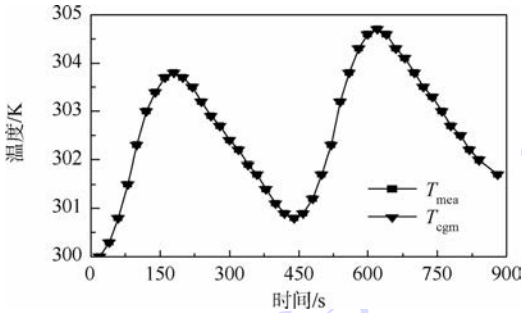
图 2 数值试验 1 的温度反演值与测量值比较
