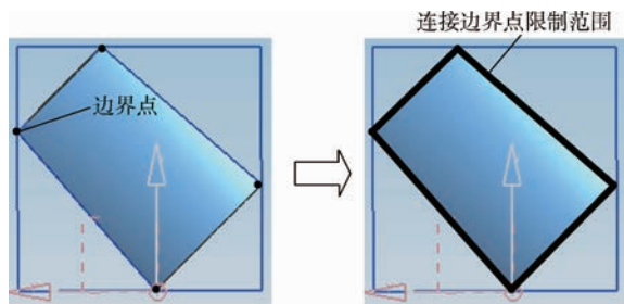
图 12 采用边界点约束可敷设区示意图
