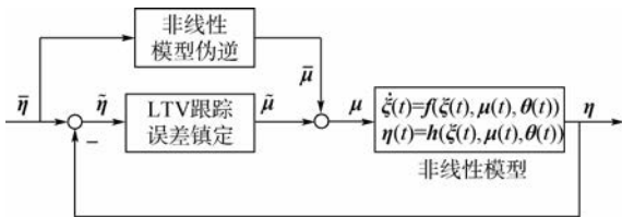
图 2 TLC 概念图 Fig. 2 Conceptual configuration of TLC
