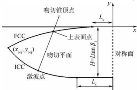
图 5 吻切锥乘波体 ICC 和 FCC 曲线定义
