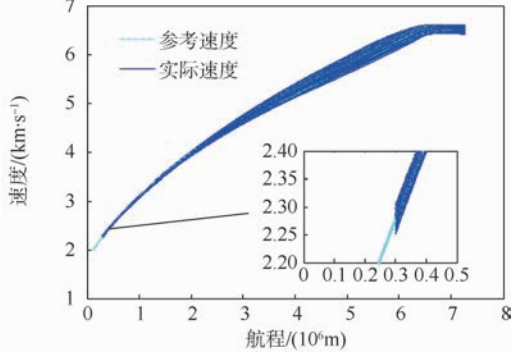
图 6 航程速度剖面的速度跟踪 Fig. 6 Velocity tracking in range-velocity profile
