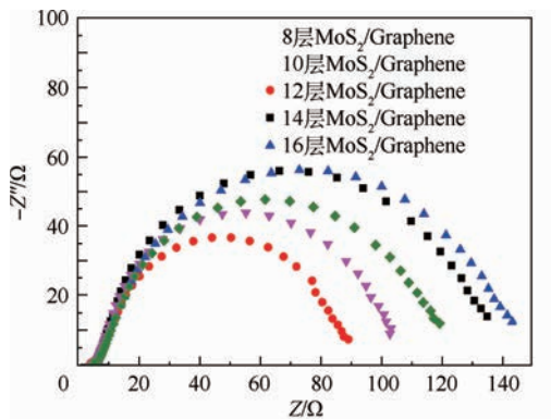
(b) 不同旋涂层数的 \text{MoS}_2/\text{Graphene} 的电化学阻抗图谱
