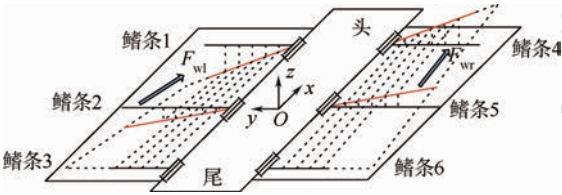
图 6 胸鳍摆动中心偏置示意图 Fig. 6 Oscillating center bias schematic of pectoral fins
