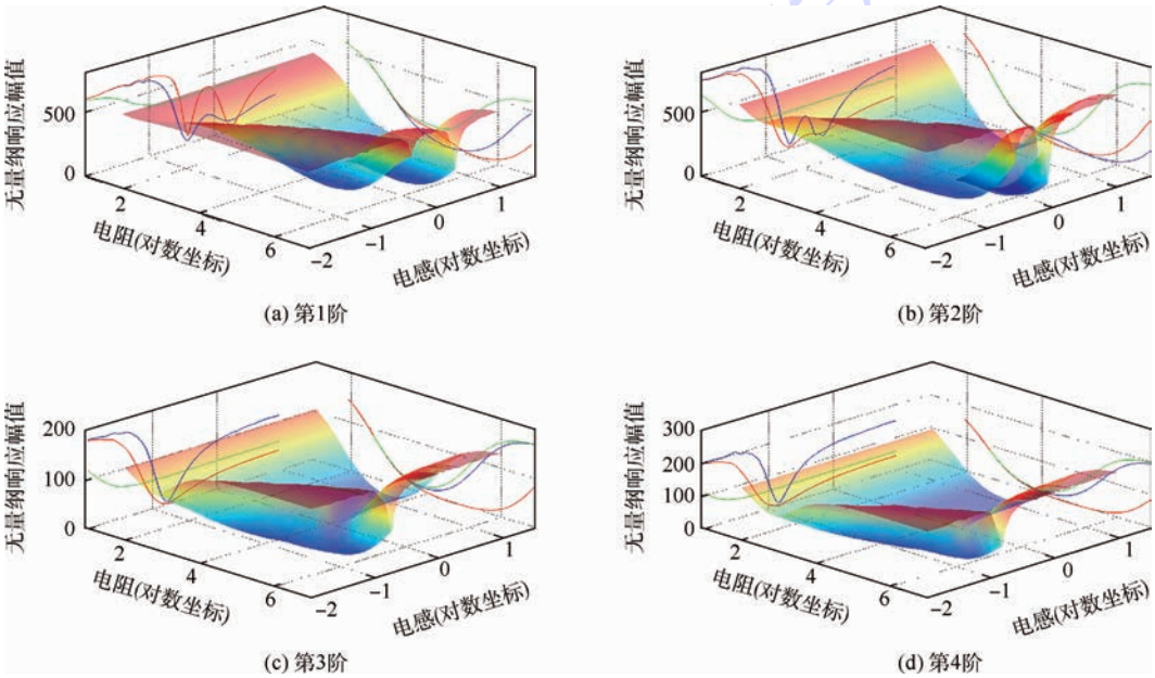
图 9 电感及电阻对共振峰值的影响(LR-PEM)
