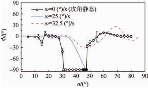
图 7 不同拉起速度时摇摆运动随攻角变化曲线对比
