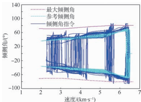
图 8 倾侧角控制历程
