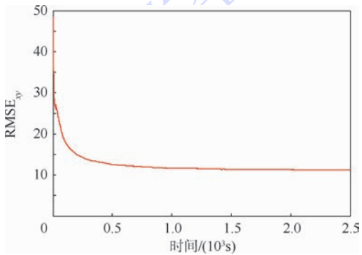
图6 目标位置估计的均方根误差
