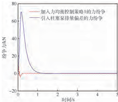
图 6 引入柱塞泵排量偏差力纷争时
