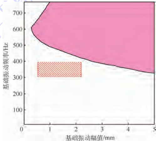
图 12 调整内径后的失效区域图 Fig. 12 Failure area chart after inner diameter's optimization
