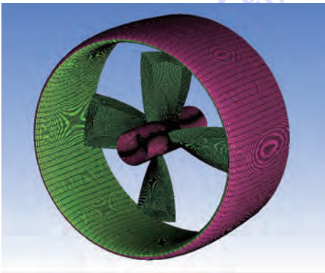
图 4 导管桨表面网格划分
