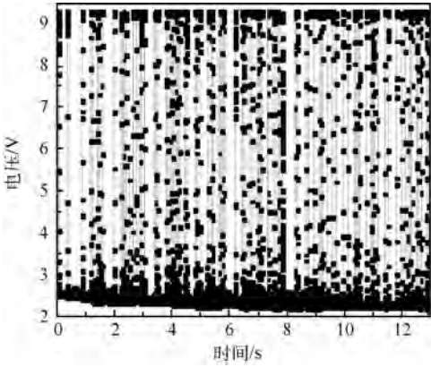
图 4 光纤探针信号时间序列
