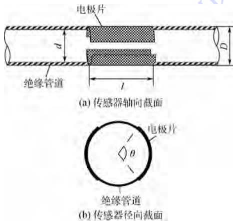
图 5 传感器基础模型截面结构
