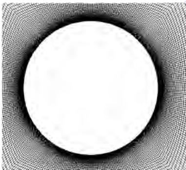
图 3 圆柱表面附近网格示意图
