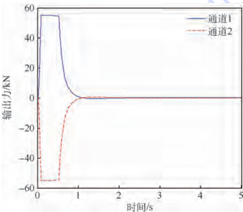
图 2 主动/主动模式下的力纷争
