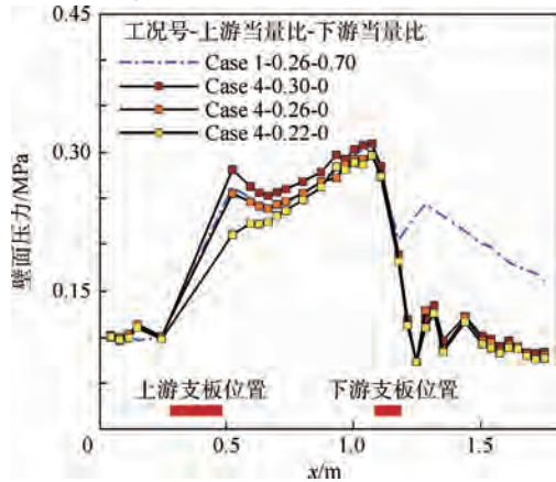
图 8 Case 4 和 Case 1 不同上游当量比壁面压力分布 Fig. 8 Wall pressure distribution of Case 4 and Case 1 with different upstream equivalence ratios
