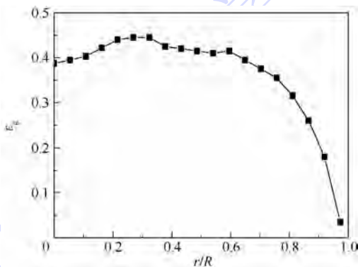
图9 费托合成反应器中气含率径向分布
