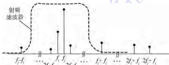
图 2 射频滤波器的频率筛选特性
