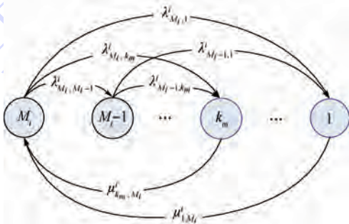
图 1 部件的 Markov 模型
