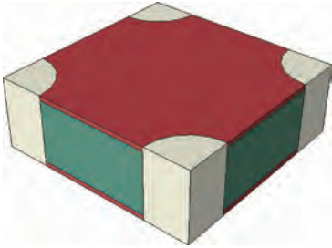
图 7 缎纹编织简化单元有限元模型
