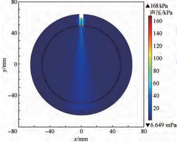
图 5 30 电极时超声场分布
