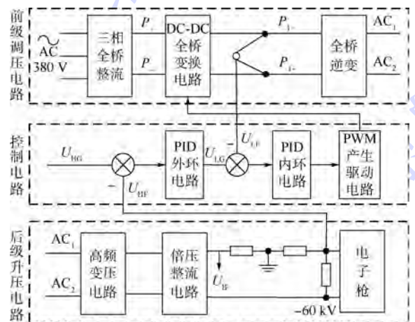
图 1 电子束焊机高压电源整体结构设计方案 P_+ —三相整流输出正极; P_- —三相整流输出负极; P_{1+} —DC-DC 全桥变换器输出正极; P_{1-} —DC-DC 全桥变换器输出负极; AC_1 —全桥逆变输出交流电压第一相; AC_2 —全桥逆变输出交流电压第二相; U_{HG} —高压外环给定电压; U_{HF} —高压外环反馈电压; U_{LG} —高压内环给定电压; U_{LF} —高压内环反馈电压; U_F —束流反馈电压。
