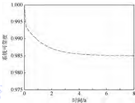
图3 系统可靠度与时间的关系
