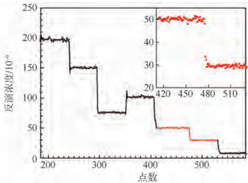
图 4 实验室 SO 2 标气测量结果 Fig. 4 Standard SO 2 measurement result in laboratory
