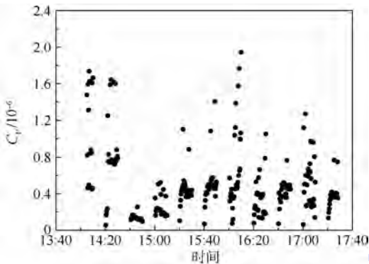
图8 除雾器出口液滴颗粒体积浓度
