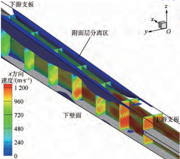
图 15 数值模拟边界层分离区
