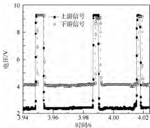
图 7 双光纤探针信号时间序列
