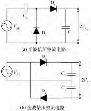
图 7 2 种倍压整流电路拓扑
