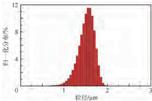
图10 某时刻液滴颗粒粒径分布
