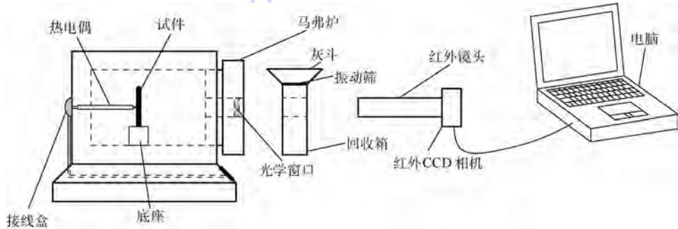
图 2 金属壁面红外测温实验系统示意图
