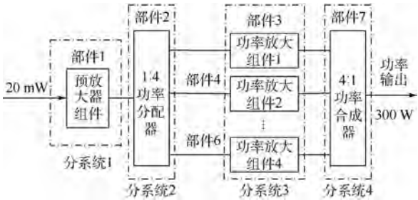
图 2 某型雷达功率放大系统
