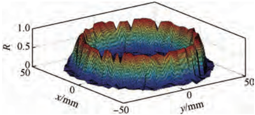
图 8 管道内电学灵敏度分布
