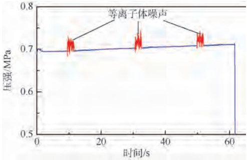
图 7 燃气发生器模拟器中的压力曲线
