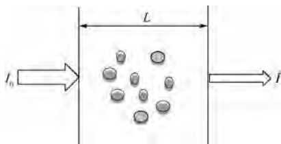
图 1 朗伯比尔定律示意图
