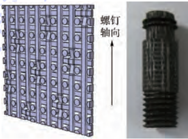
图3 缎纹编织碳/碳复合材料试验件加工方向示意图
