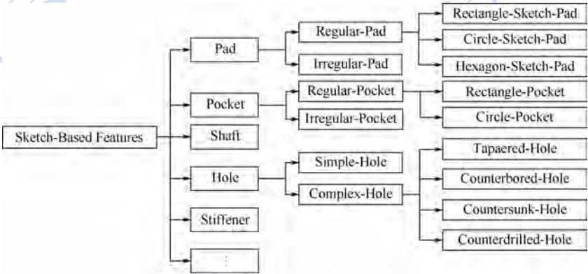
图 4 基于草图的特征本体分类及数据属性
