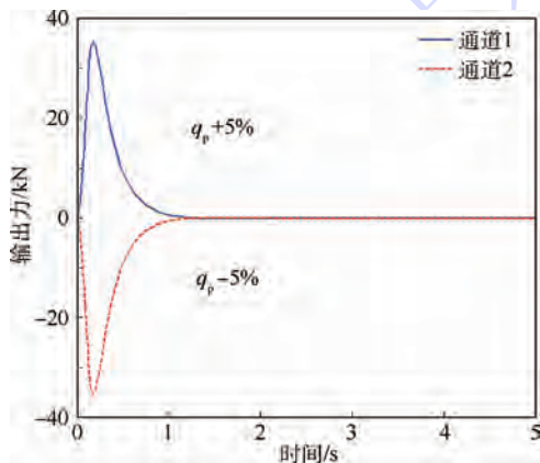
图 4 柱塞泵排量偏差造成的力纷争
