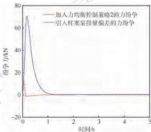
图 9 引入柱塞泵排量偏差力纷争时无力均衡控制策略 2 的仿真结果
