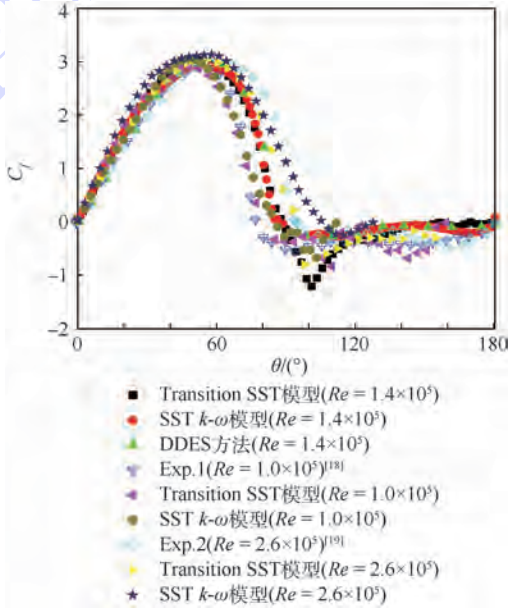
图 5 在亚临界区圆柱表面时均摩擦力系数 C_f 分布曲线
