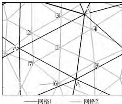
图1 重叠区域网格尺寸不匹配
