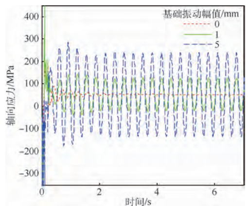
图 3 应力敏感截面上最大应力响应
