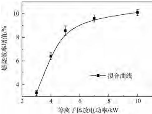
图 9 等离子体放电功率对多组分燃气在发动机中燃烧效率的影响
