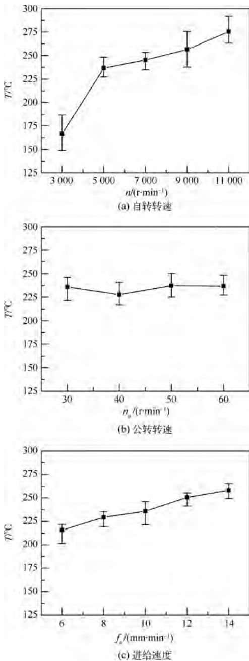
图5 自转转速、公转转速及进给速度对切削温度的影响
