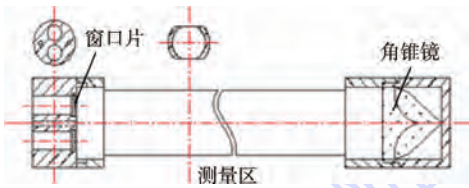
图 2 光学探针结构图 Fig. 2 Schematic of optical probe structure
