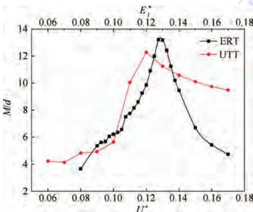
图 12 超声探头相对直径与电极相对宽度对超声敏感场 M/d 的影响
