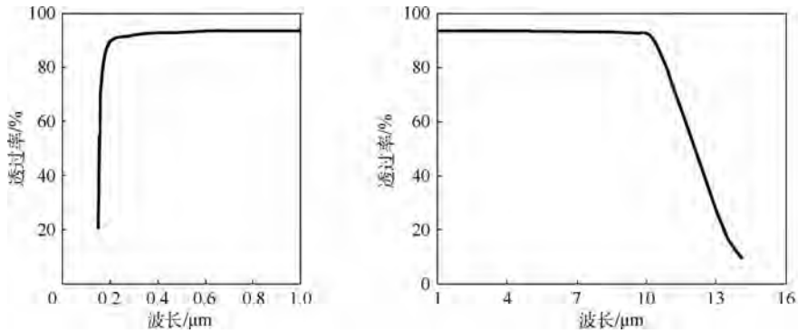
图3 光学窗口的透过率曲线
