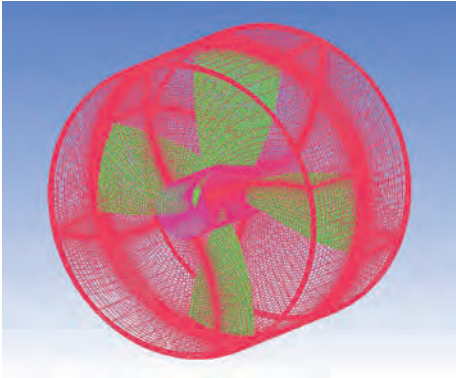
图 2 旋转域网格示意图
