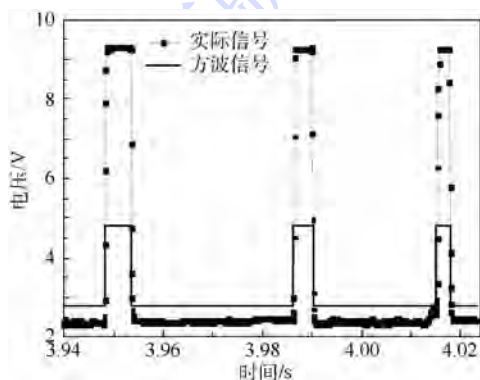
图 5 局部放大后的光纤探针信号
