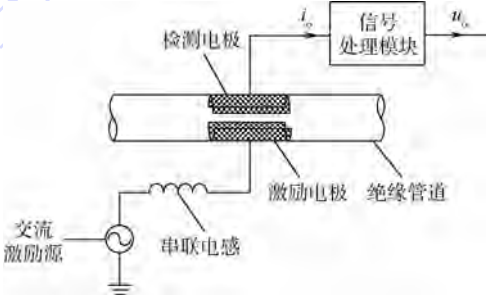
图 3 径向两电极传感器结构
