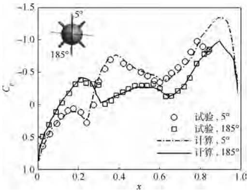
图 13 初始时刻 5^\circ 和 185^\circ 子母线压力系数分布 Fig. 13 Pressure coefficient distribution on circumferential location 5^\circ and 185^\circ at initial time
