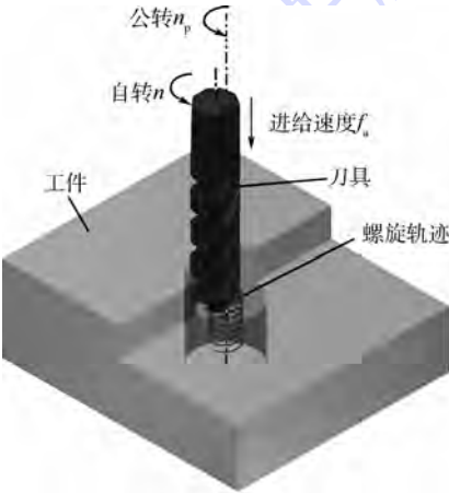
图 1 螺旋铣孔原理 Fig. 1 Principle of helical milling
