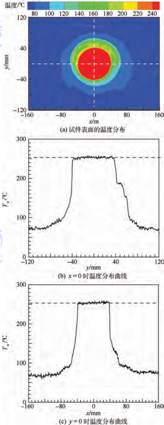
图4 红外 CCD 相机测量的温度分布
