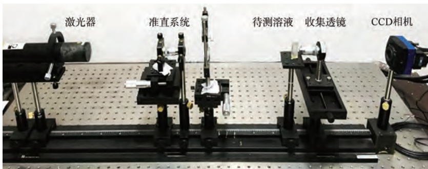
图 3 近场散射粒径测量系统实验装置图
