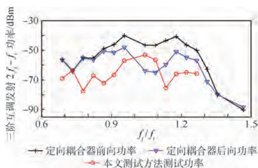
图9 f_m = 2f_j - f_i 时的互调发射测试电平
