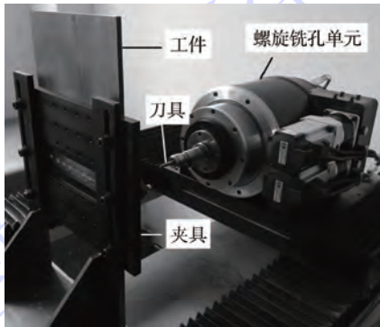
图 4 螺旋铣孔单元
