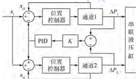
图 5 差值力补偿力均衡控制原理图
