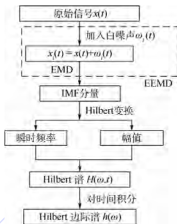
图 1 EEMD-Hilbert 谱的计算流程
