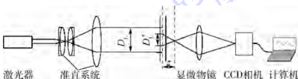
图 1 近场散射原理图
