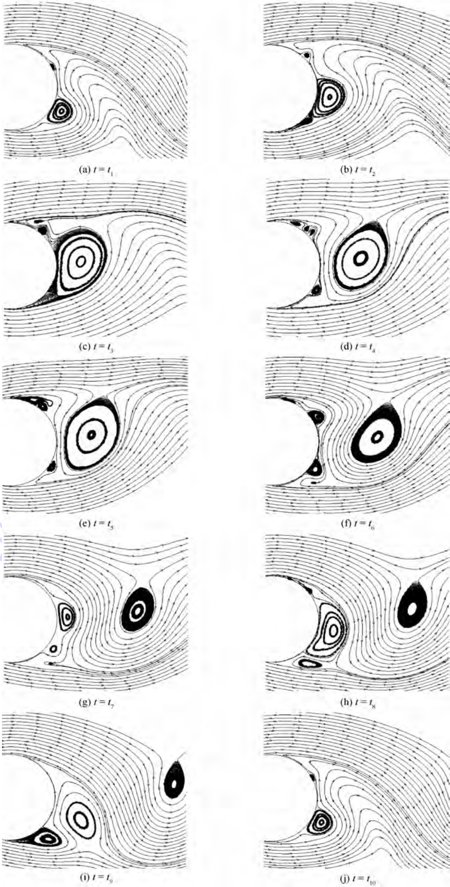
图 6 在亚临界区时采用 Transition SST 模型模拟一个周期内的流线
