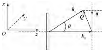
图 2 近场散射矢量图
