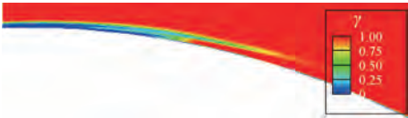
图 11 圆柱上表面间歇因子云图
