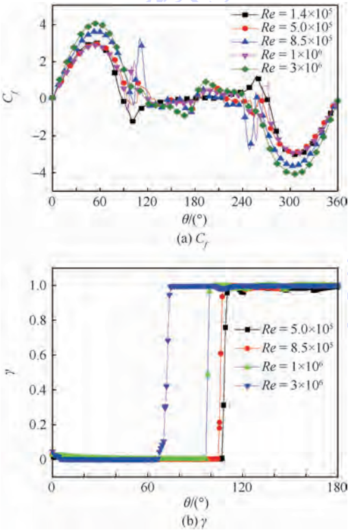
图 13 不同雷诺数下圆柱表面时均摩擦力系数 C_f 和间歇因子 \gamma 分布曲线
