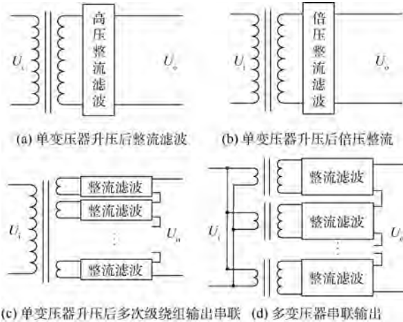
图 5 变压器主要升压方式 Fig. 5 Common methods of boosting transformer
