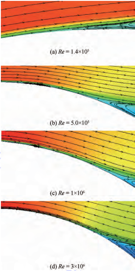
图 14 不同雷诺数下圆柱上表面附近局部流场速度分布云图和流线图
