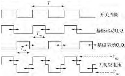
图 3 IGBT 全桥逆变电路工作原理示意图 Fig. 3 Fundamental diagram of IGBT full-bridge inverter
