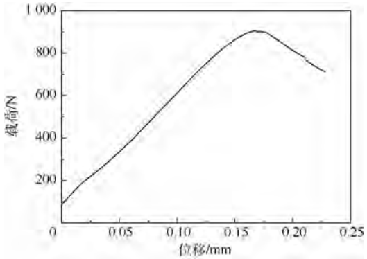
图 5 试验载荷-位移曲线 Fig.5 Force-displacement curve of test
