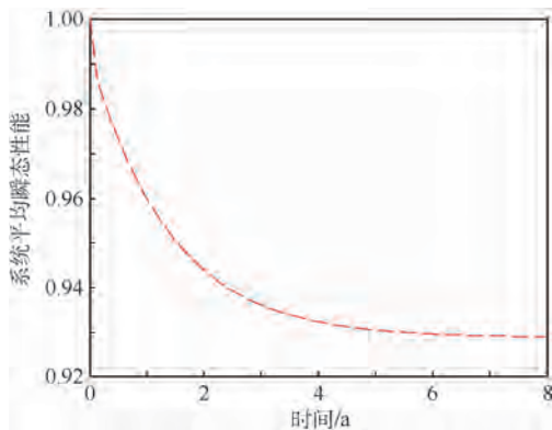
图4 系统平均瞬态性能与时间的关系
