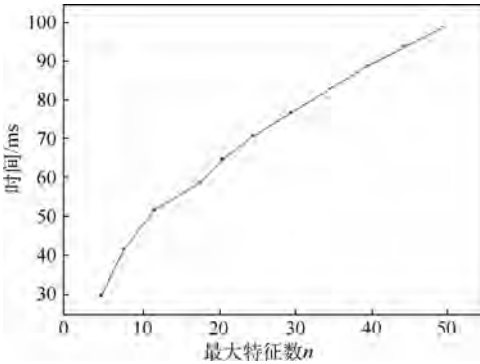
图 16 时间与最大特征数 n 的关系
