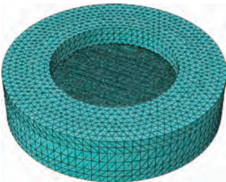
图 9 螺牙及螺母有限元网格
