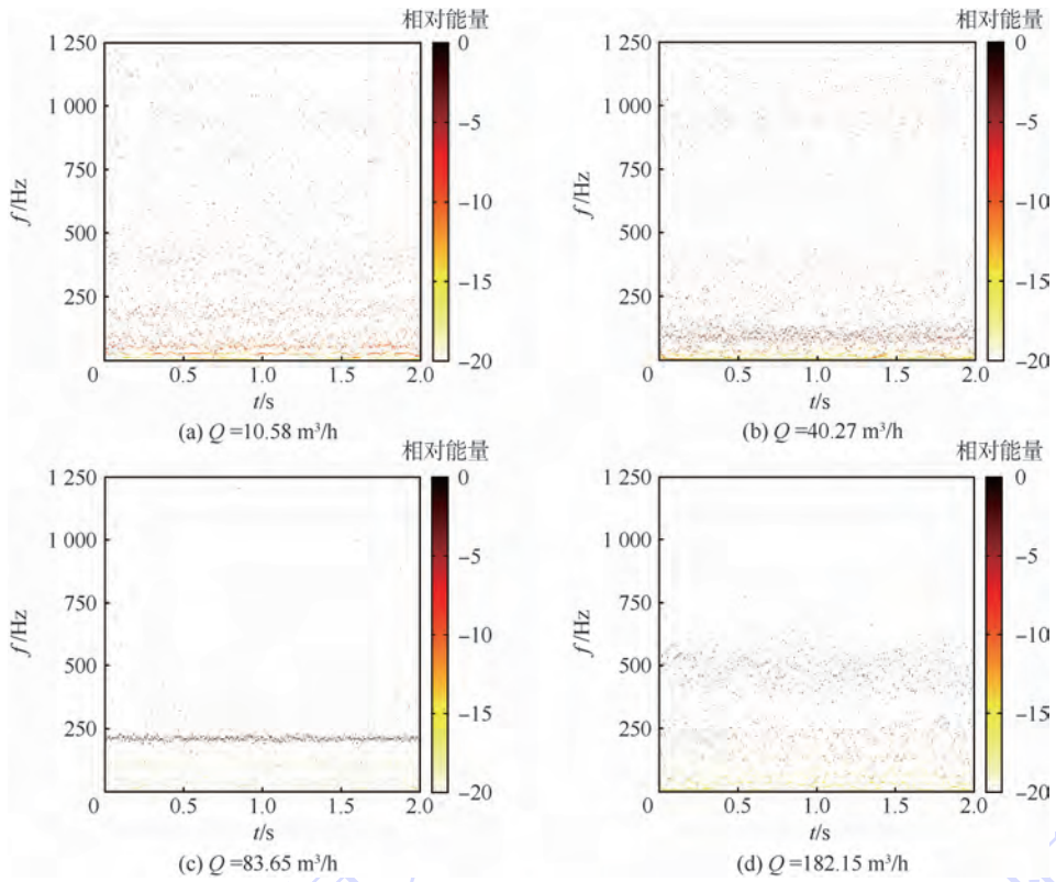
图 4 不同流量下尾迹的 Hilbert 谱 Fig.4 Hilbert spectra of wake at different flow rates
