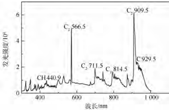
图 5 等离子体炬的发射光谱
