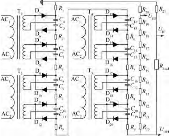
图 6 后级高压电路拓扑
