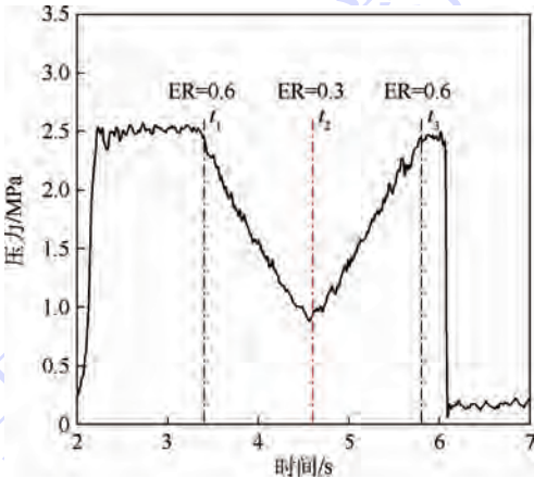
图 9 Case 5 文氏管后压力随时间的变化 Fig. 9 Case 5 time history of pressure after venturi
