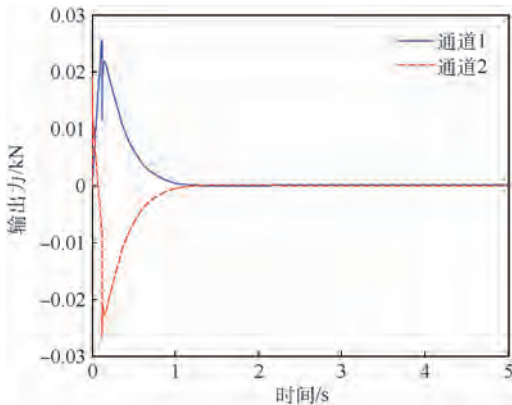
图 3 流量补偿后的力纷争现象
