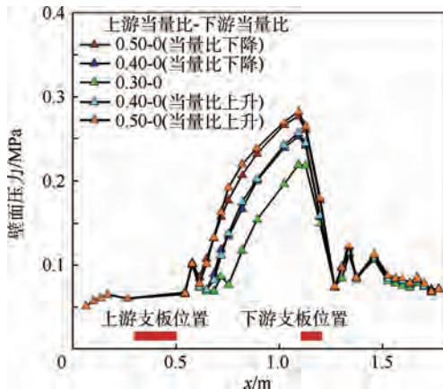
图 17 Case 7 不同上游当量比壁面压力分布 Fig. 17 Wall pressure distribution of Case 7 with different upstream equivalence ratios
