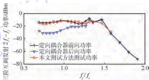
图8 f_m = 2f_i - f_j 时的互调发射测试电平
