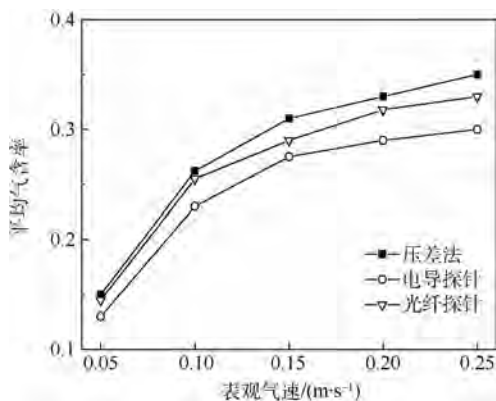
图 6 不同方法所得平均气含率的比较
