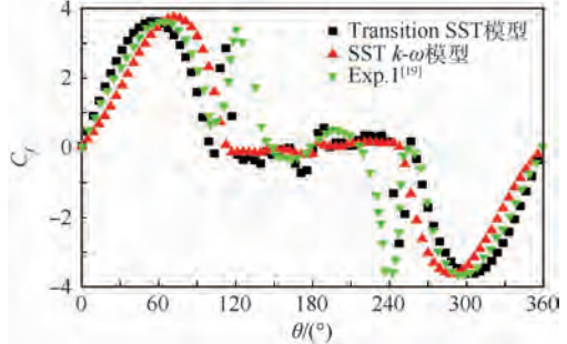
图 8 在临界区圆柱表面时均摩擦力系数 C_f 分布曲线 Fig. 8 Distribution curves of time-averaged friction coefficient C_f on cylindrical surface in critical region
