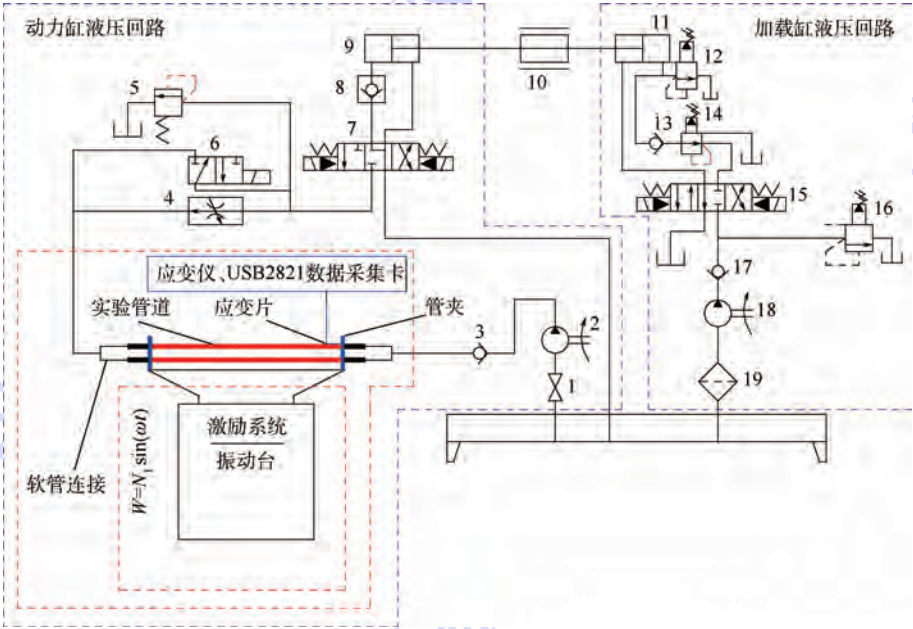
1—油源开关; 2—变量泵; 3,13,17—单向阀; 4—调速阀; 5,12—电磁溢流阀; 6—换向阀; 7,15—电磁换向阀; 8—液控单向阀; 9—动力液压缸; 10—惯性负载; 11—加载液压缸; 14—电磁减压阀; 16—溢流阀; 18—定量泵; 19—过滤器。
