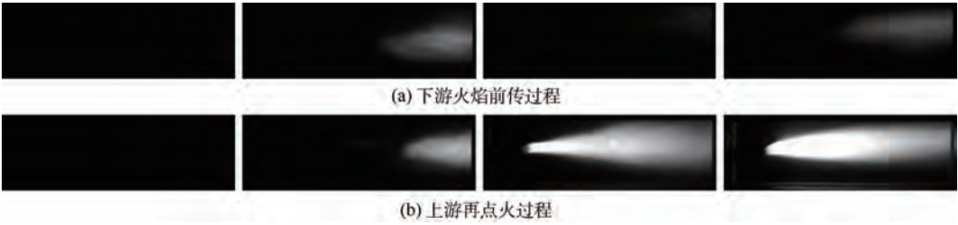
图 14 上游火焰瞬态图像 ( \Delta t = 0.5\text{ ms} )
