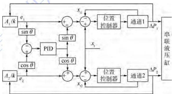
图 8 交叉耦合力均衡控制原理图
