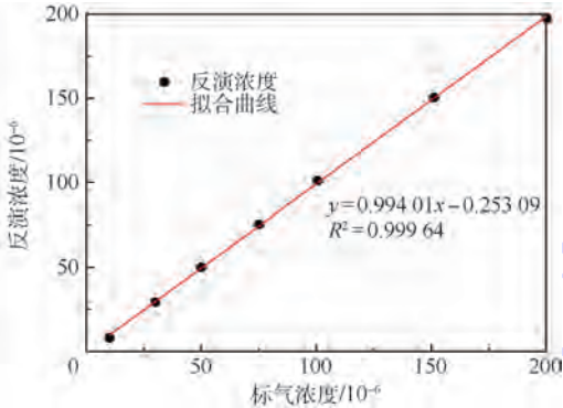
图 5 SO 2 标气测量结果
