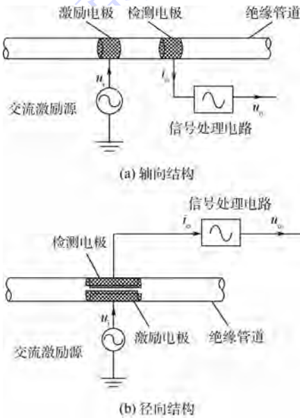
图 1 C 4 D 传感器典型结构
