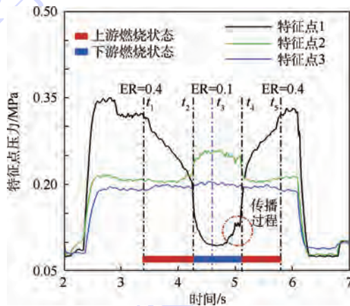
图 13 Case 6 特征点压力随时间的变化 Fig. 13 Time history of feature points pressure of Case 6
