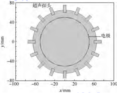
图 6 16 电极、16 超声探头结构
