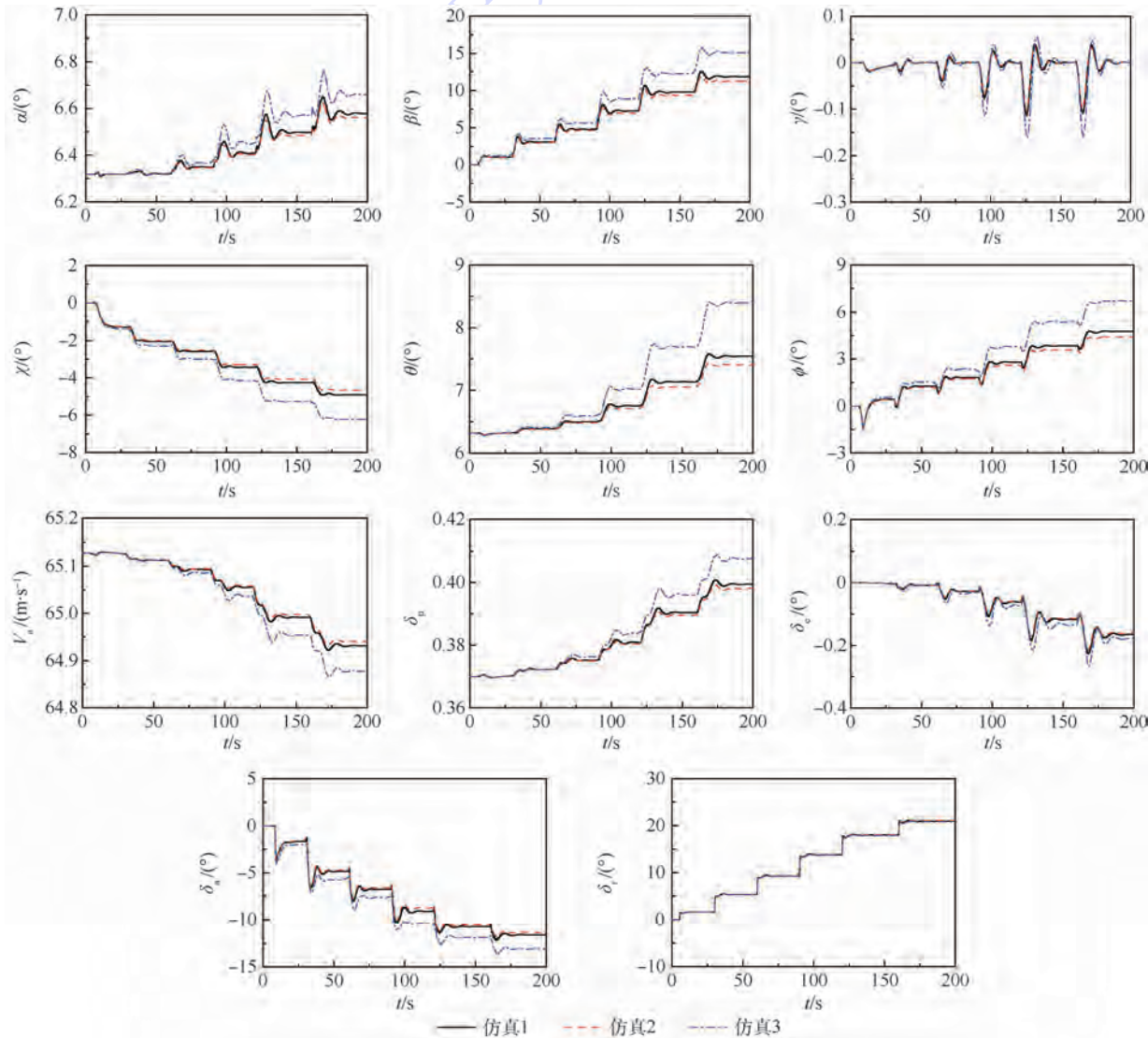
图 5 横航向静稳定性评估仿真结果
