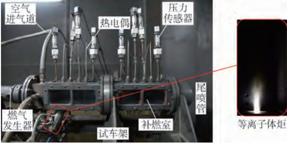
图 4 等离子体炬放电照片
