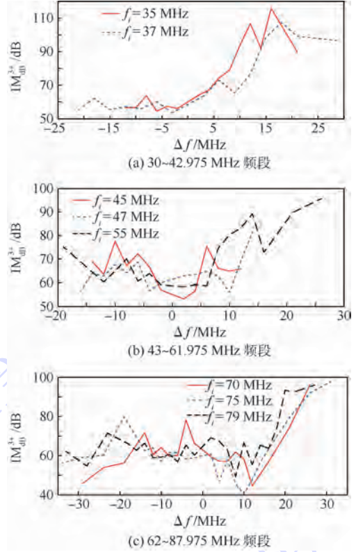
图 11 f_m = 2f_j - f_i 时不同工作频段的互调抑制比 IM_{dB}^{3+}
