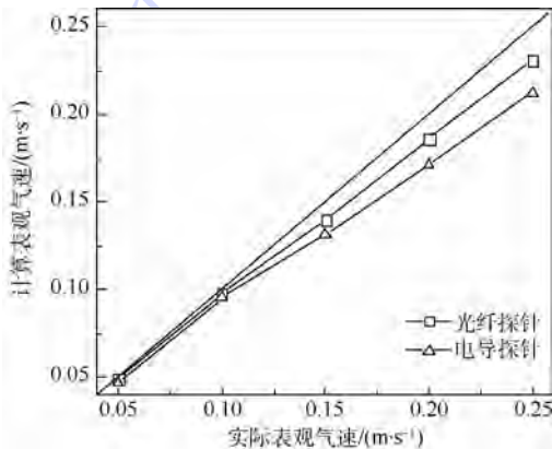
图8 探针法计算得到的表观气速与实际表观气速对比
