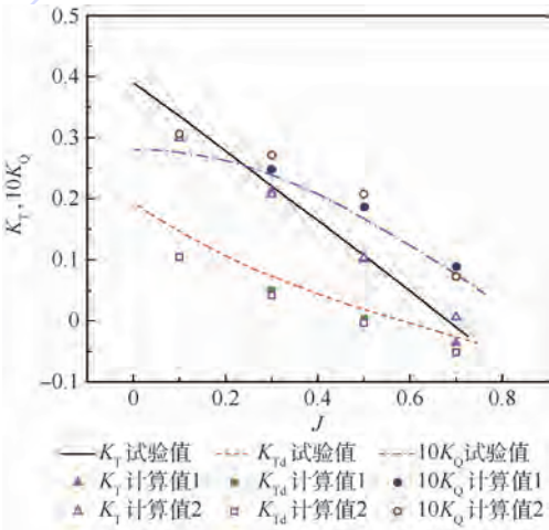
图 5 JD7704 + Ka4-5508 型导管桨敞水特性的计算值与试验值比较
