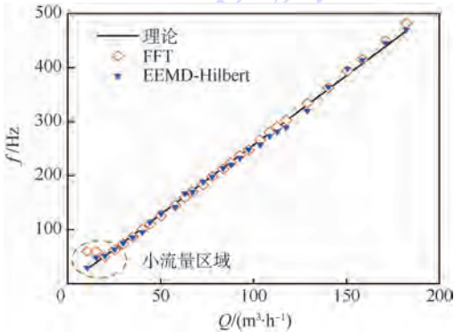
图 5 尾迹波动的流量与涡街频率的关系 Fig.5 Wake fluctuation flow rates versus frequencies
