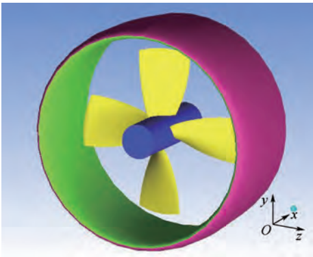
图 1 导管桨三维模型
