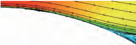
图 12 圆柱上表面速度云图和流线图
