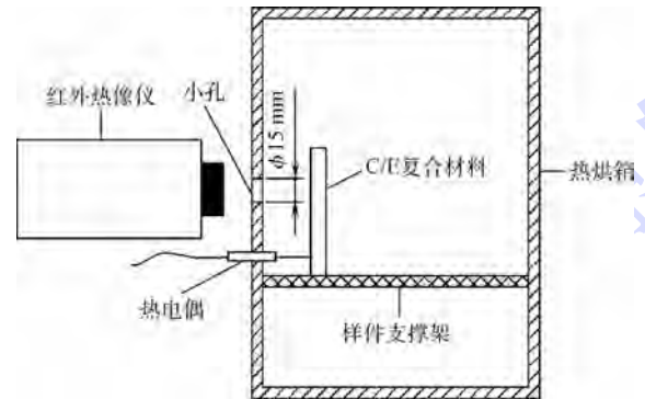
图 3 红外热像仪标定方法
