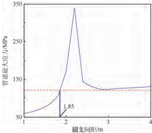
图 10 不同固支间距下管道最大应力 Fig. 10 Maximum pipe stress under different support spans
