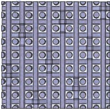
图1 8枚缎纹编织复合材料单胞
