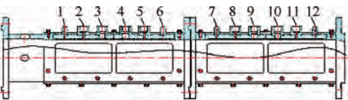
图 3 补燃室不同截面的测量装置
