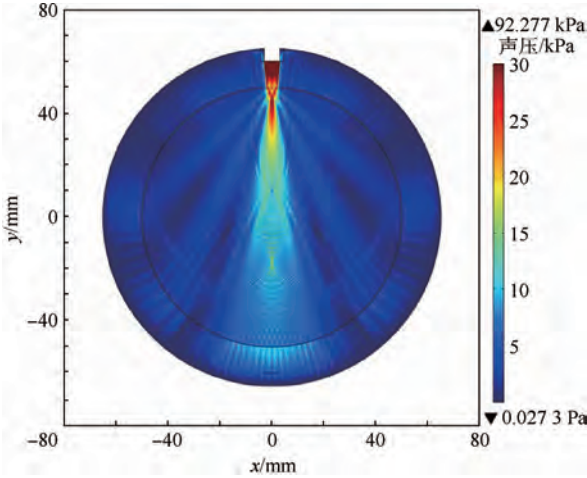
图 3 无电极时超声场分布
