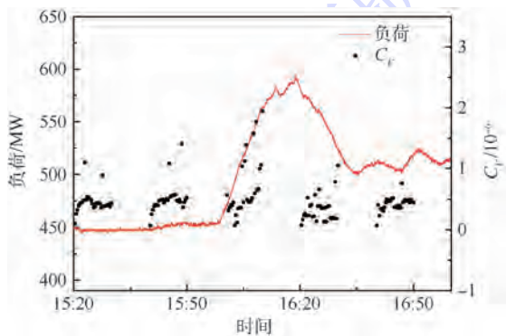
图9 液滴颗粒浓度与锅炉负荷
