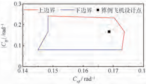
图 8 C_{n\beta} 和 |C_{l\beta}| 的可行域
