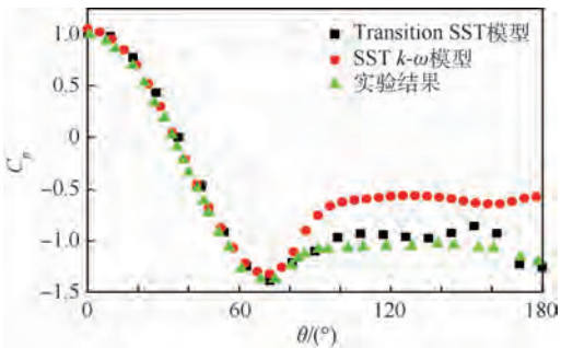
图 4 在亚临界区圆柱表面时均压力系数 C_p 分布曲线
