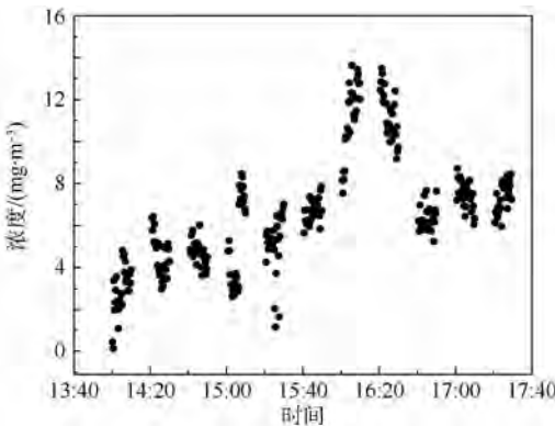
图 7 实验测得烟气中 SO 2 浓度
