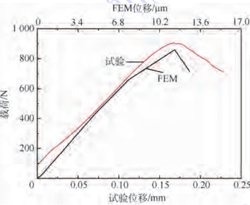
图 12 试验和有限元方法载荷-位移曲线 Fig. 12 Force-displacement curves of test and FEM
