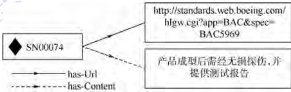
图 12 工程注释项本体结构 Fig. 12 Engineering note item ontology structure
