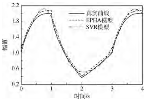
图 5 EPHA 模型与 SVR 模型系统行为曲线 Fig.5 System behavior curves of EPHA model and SVR model
