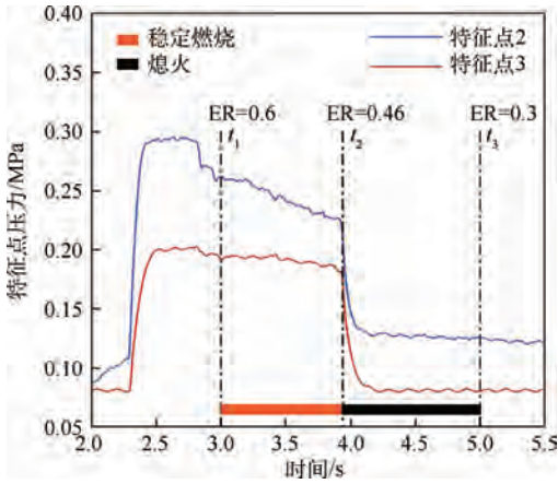
图 6 Case 2 特征点压力随时间的变化 Fig. 6 Time history of feature points pressure of Case 2
