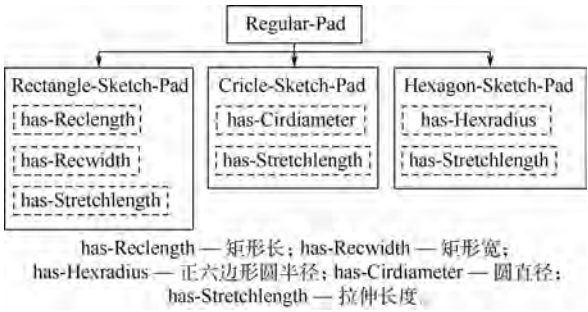
图 5 规则草图凸台特征数据属性
