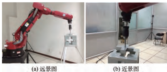
图 1 实体机械臂对接场景
