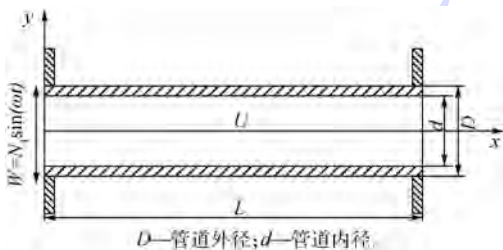
图1 管道理论模型
