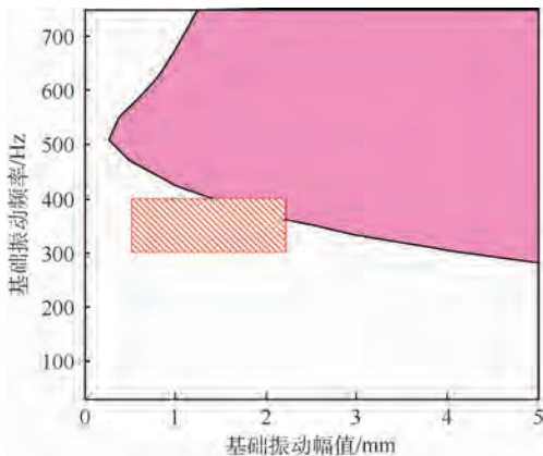
图 11 不同基础振动参数下的失效区域 Fig. 11 Failure area of different foundation vibration parameters
