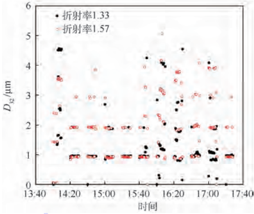
图 6 折射率为 1.33 和 1.57 时得到的液滴索太尔平均直径
