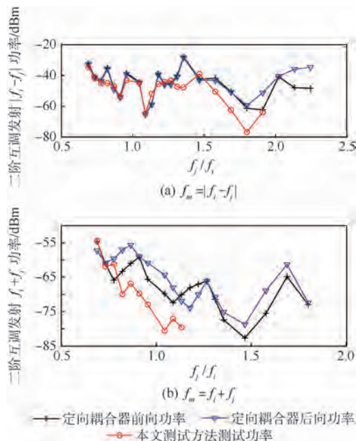
图7 f_m = |f_i - f_j| 和 f_m = f_i + f_j 时的互调发射测试电平
