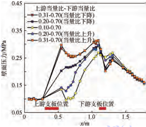
图 16 Case 6 不同上游当量比壁面压力分布
