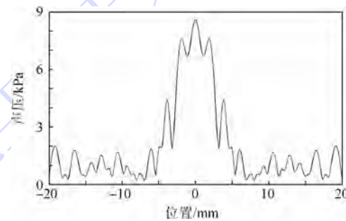
图2 声压强度分布
