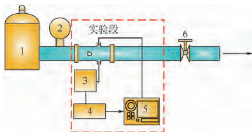
1—钟罩式气体流量标准装置; 2—流量显示装置; 3—差压传感器; 4—信号调理板; 5—数字示波器; 6—球阀。
