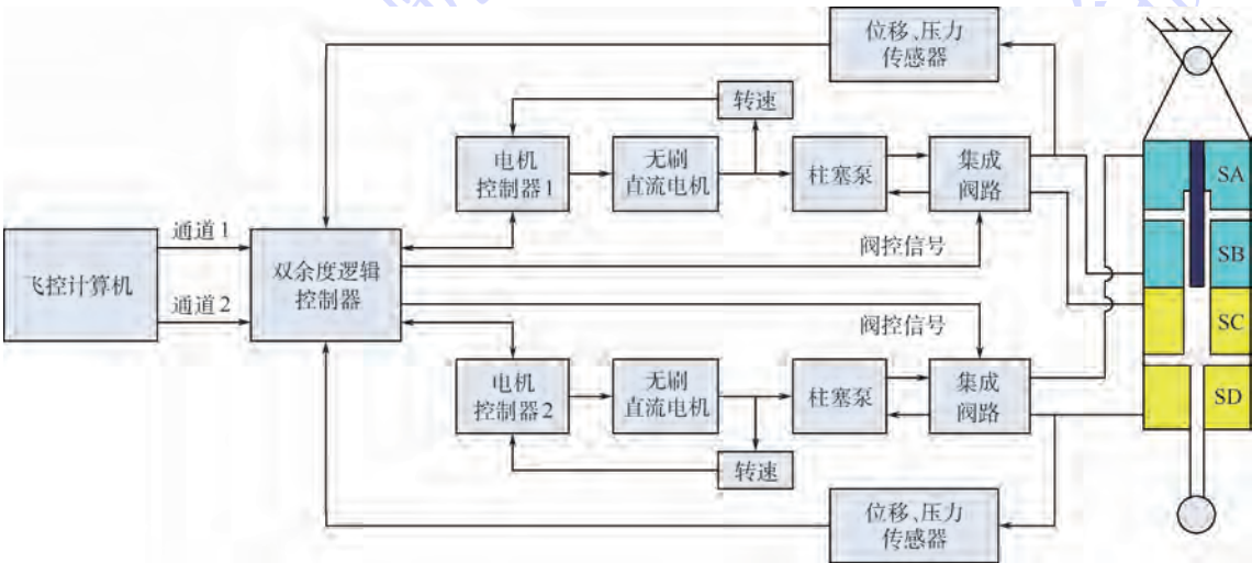
图 1 DREHA 系统结构原理图 Fig. 1 Schematic diagram of DREHA system structure
