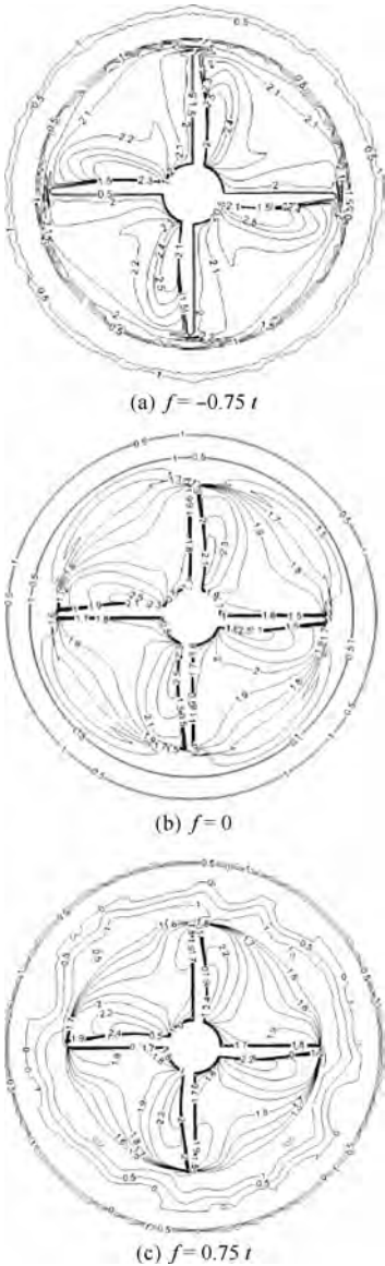
图 14 f = -0.75 t f = 0 和 f = 0.75 t 时 导管桨 x/R = 0 处轴向速度分布
