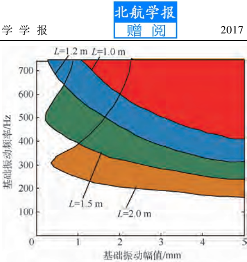
图 8 不同固支间距下管道失效区域图 Fig. 8 Area chart of pipe failure under different support spans
