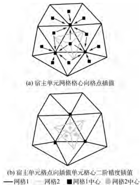
图4 第2类情况插值示意图
