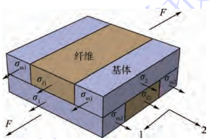
F—碳布单元受力; \sigma_{f1} —上层纤维束 1 方向正应力; \sigma_{f2} —下层纤维束 2 方向正应力; \sigma_{m1} 、 \sigma_{m2} —上层和下层基体 1 方向正应力; \sigma_{m2} 、 \sigma_{m2} —下层和上层基体 2 方向正应力。
