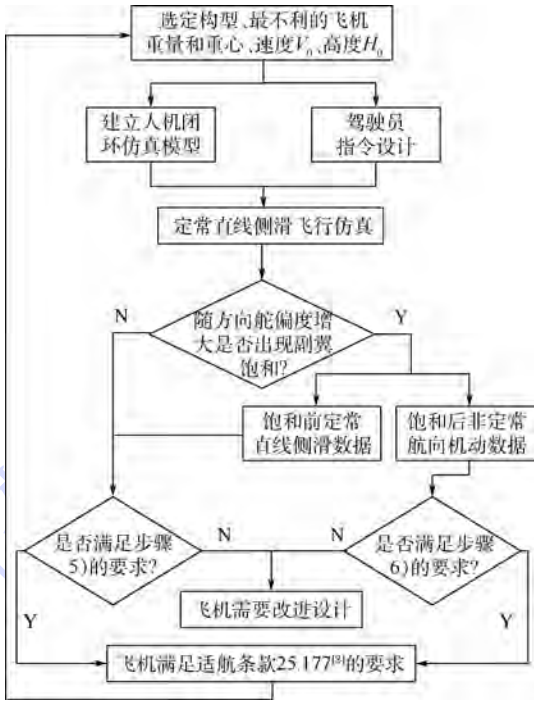
图 4 仿真流程
