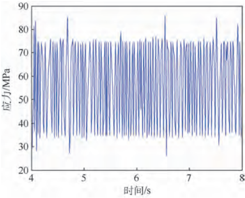
图 13 优化后应力敏感截面上最大应力响应
