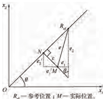
图 7 交叉耦合控制
