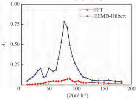
图 6 尾迹波动的流量与能量比的关系 Fig. 6 Wake fluctuation flow rates versus energy ratio
