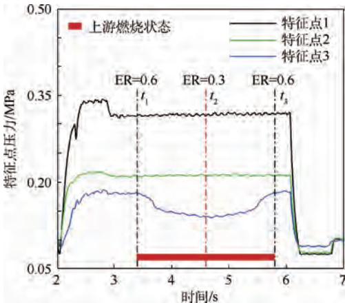
图 10 Case 5 特征点压力随时间的变化 Fig. 10 Case 5 time history of feature points pressure
