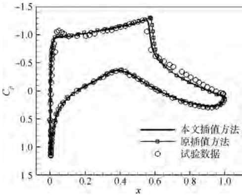
图 8 翼面压力系数分布 Fig. 8 Pressure coefficient distribution on wing surface
