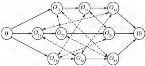
图 1 析取图模型
