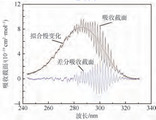
图 3 实验室标定得到的 SO 2 吸收截面及处理结果 Fig. 3 SO 2 absorption cross sections obtained from laboratory calibration and results
