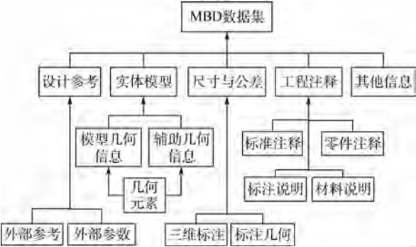
图 1 MBD 数据集
