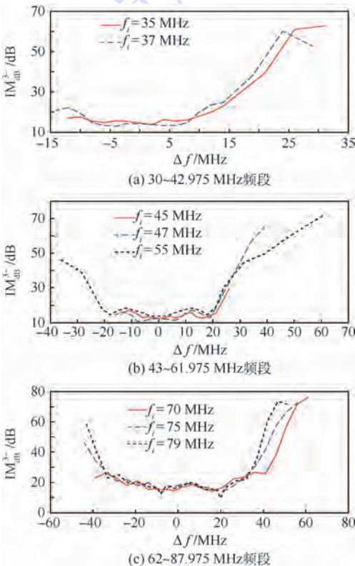
图 10 f_m = 2f_i - f_j 时不同工作频段的互调抑制比 IM_{dB}^{3-}
