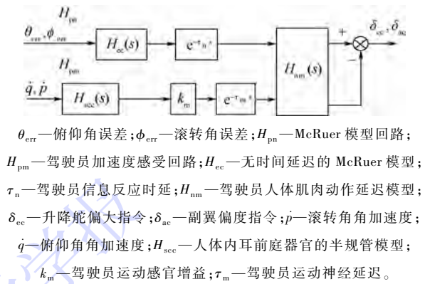
图 3 Hosman 驾驶员模型
