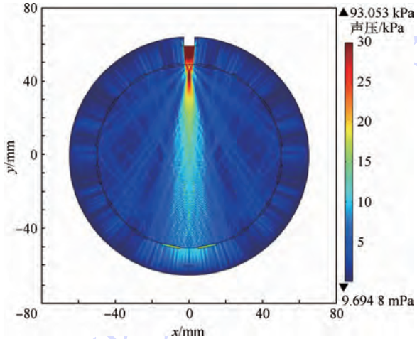
图 4 16 电极时超声场分布
