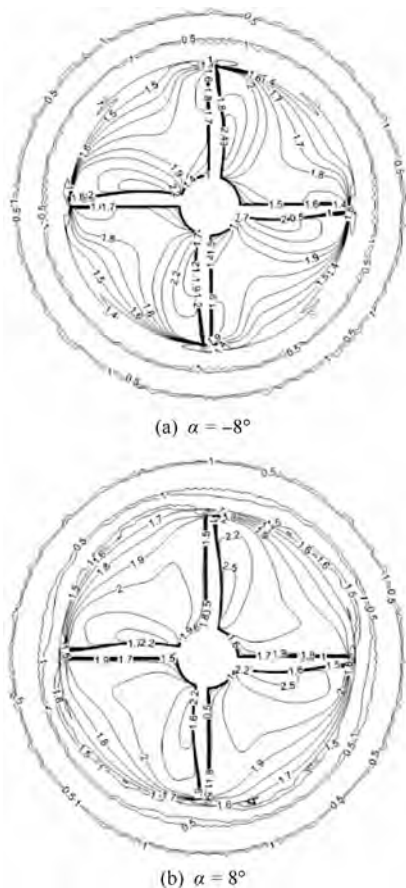
图 22 攻角为 -8^\circ 和 8^\circ 时导管桨 x/R=0 处轴向速度分布
