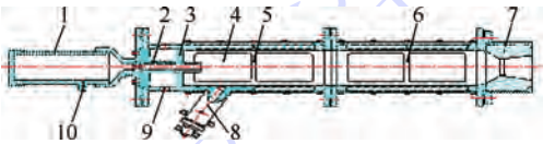
1—燃气发生器模拟器; 2—长尾管; 3—平行进气装置; 4—观察窗; 5—补燃室前端; 6—补燃室后端; 7—冲压喷管; 8—等离子体炬; 9—来流空气入口; 10—多组分燃气供给系统。
