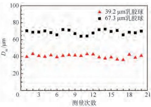
图 7 39.2 μm 和 67.3 μm 乳胶球测量结果 Fig. 7 Measurement results of 39.2 μm and 67.3 μm latex spheres
