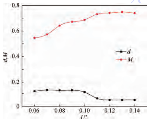
图 11 超声探头相对直径对超声敏感场平均灵敏度的影响
