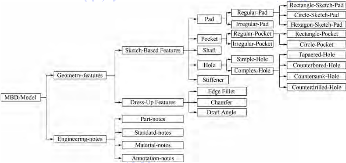
图 13 MBD 模型完整本体结构 Fig. 13 MBD model full ontology structure
